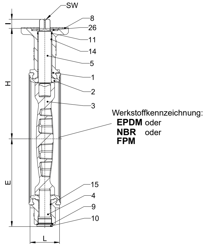
Bild 1: Absperrklappe
