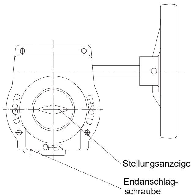
Bild 4: Getriebe
