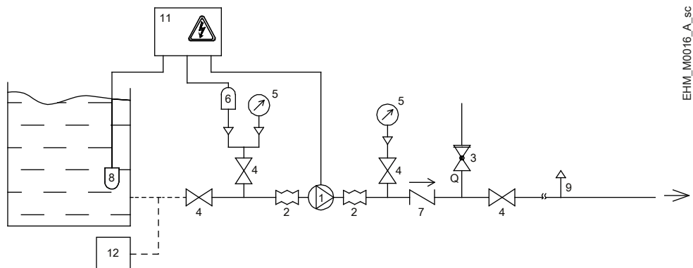
Mynd 1: Uppsetning á jákvæðum soghaus
