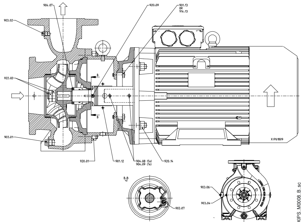
Blockerad pump med fastskruvat höljeskydd
