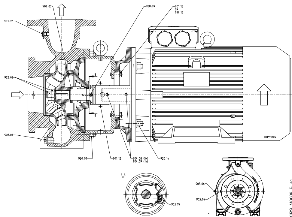
Pompe bloquée avec couvercle de carter boulonné
