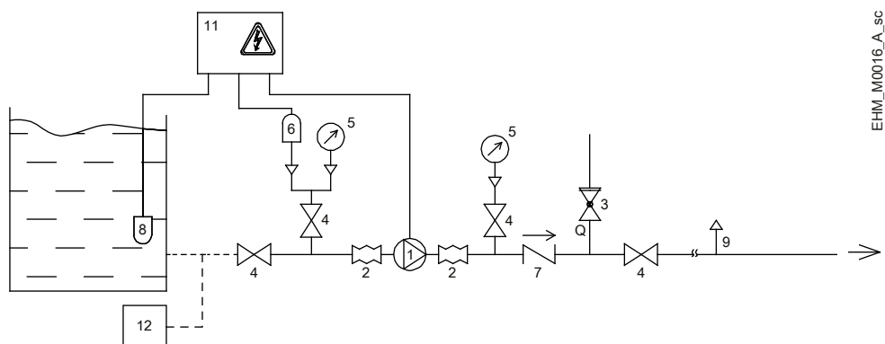
Рисунок 1: Монтаж с кавитационным запасом
