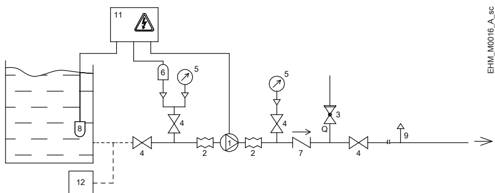
Figura 1: Installazione sottobattente
