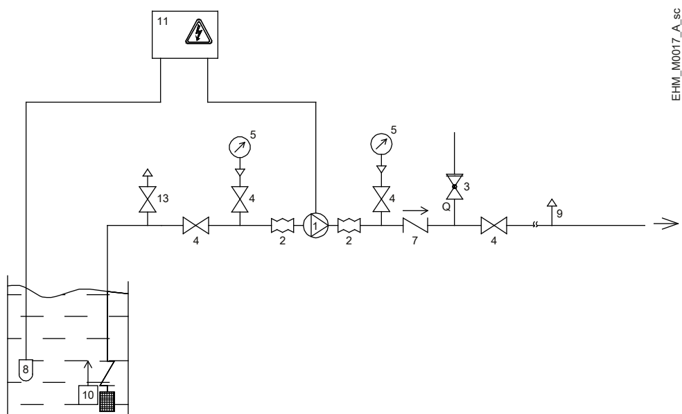
Figura 2: Installazione soprabattente
