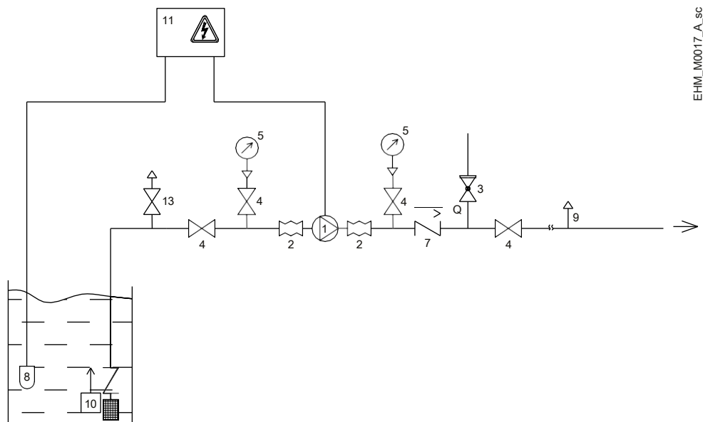
Figura 11: Schema installazione soprabattente
