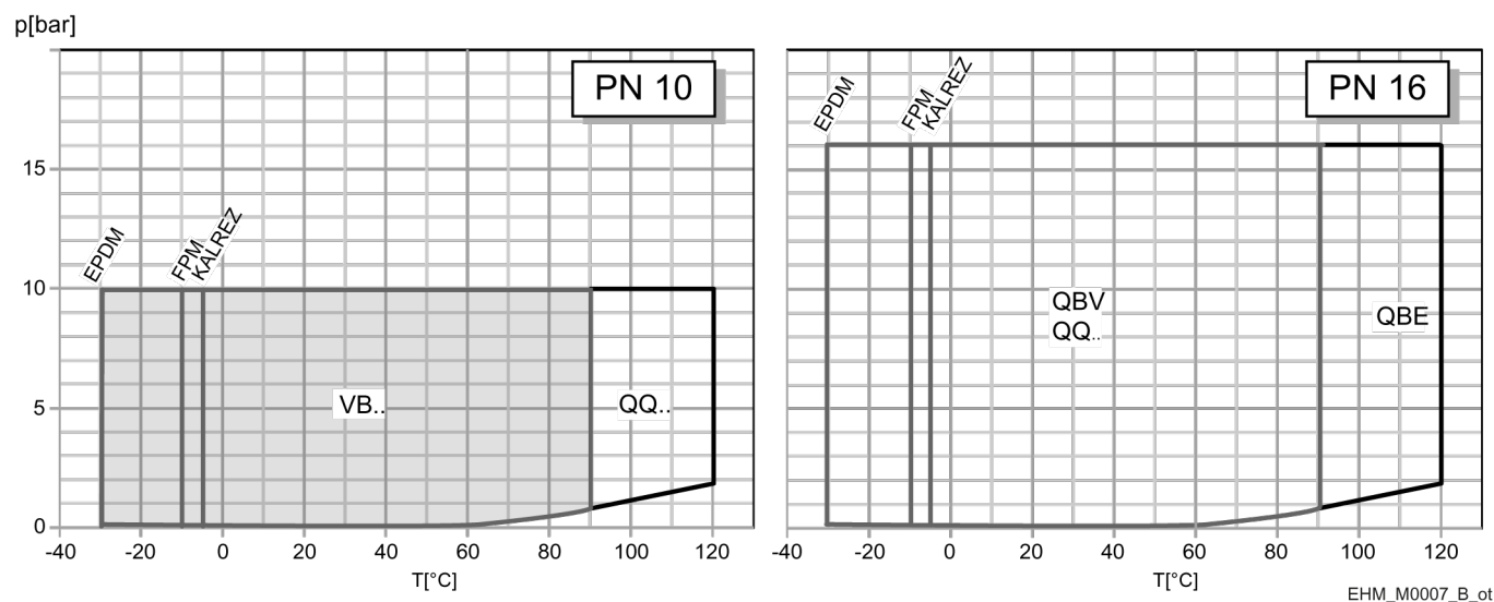
Figura 16: Diagrammi pressione-temperatura
