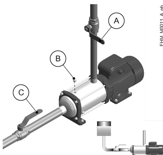
Figura 13: Adescamento installazione sottobattente
