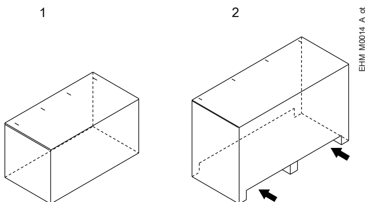
Figura 1: Punti di sollevamento del prodotto imballato
