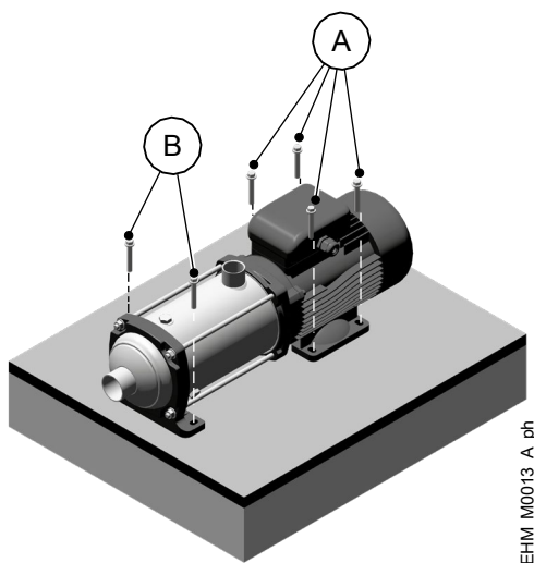
Figura 9: Fissaggio dell'unità
