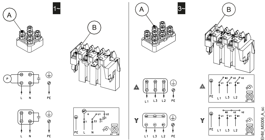
Figura 12: Collegamento elettrico e coppie di serraggio
