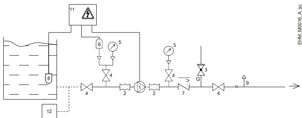
Figura 10: Schema installazione sottobattente
