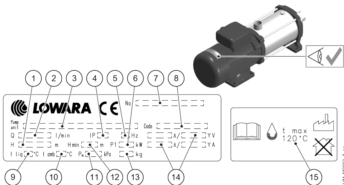
Figura 4: Targa dati
