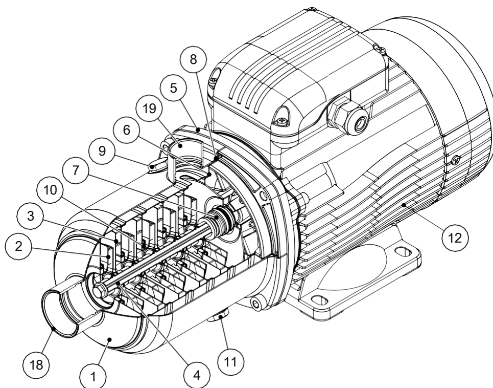
Figura 6: Elettropompa con corpo monoblocco
