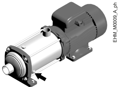
Figura 3: Tappo di scarico
