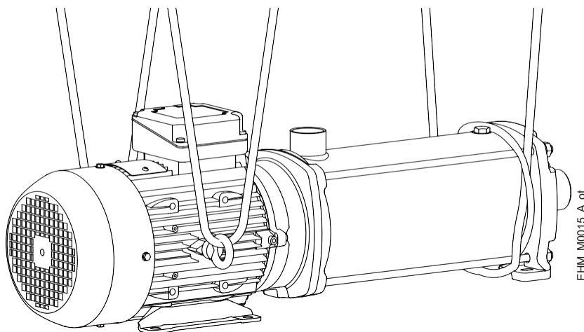
Figura 2: Sollevamento dell'unità
