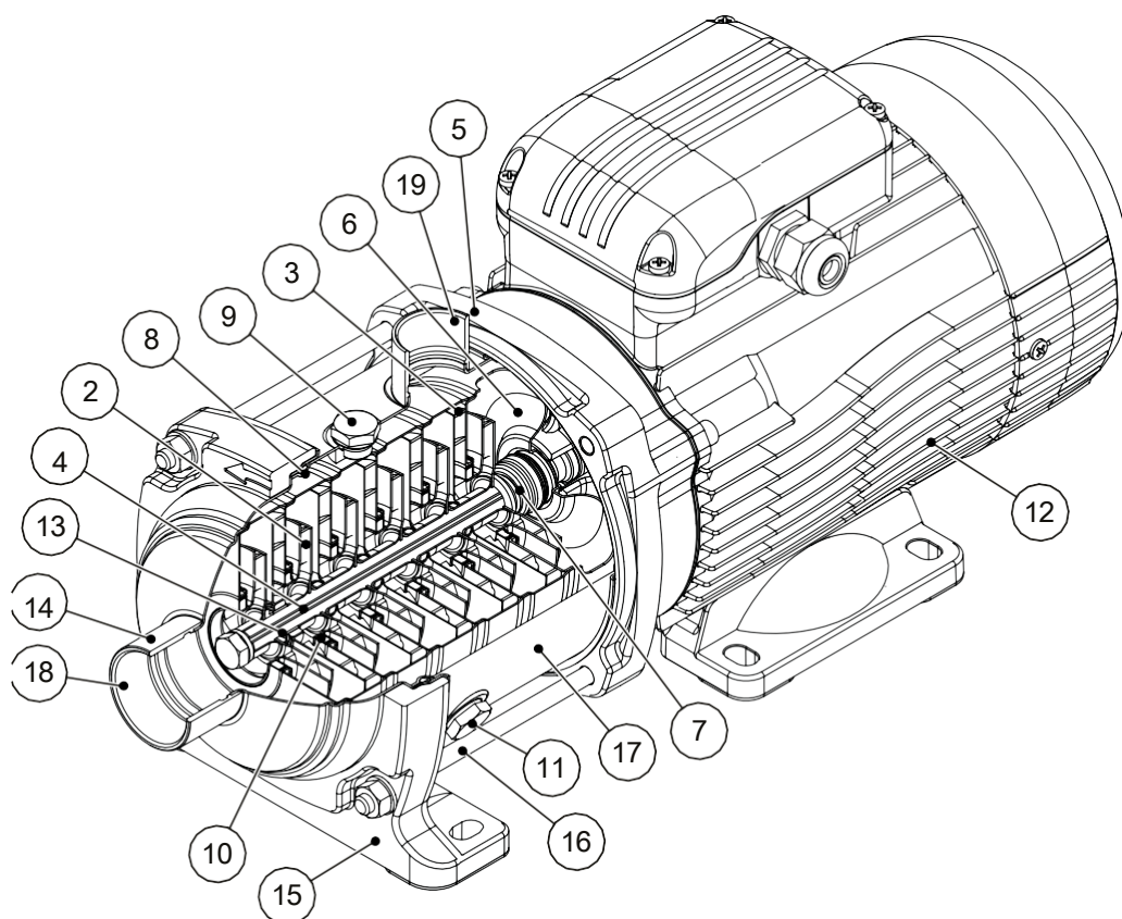
Figura 7: Elettropompa con corpo con camicia
