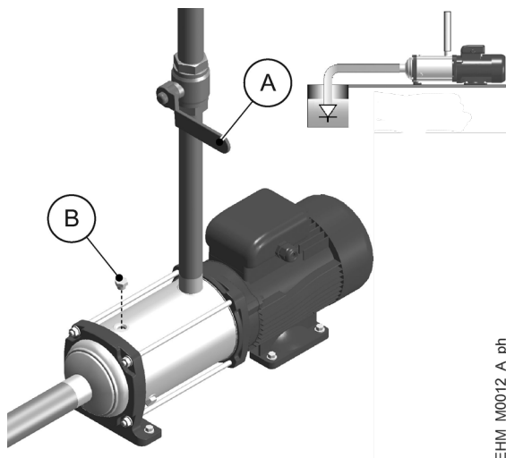
Figura 14: Adescamento installazione soprabattente
