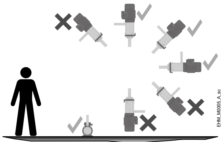
Figura 8: Posizioni dell'unità
