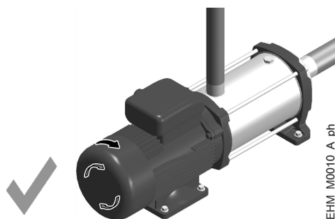
Figura 15: Senso di rotazione del motore
