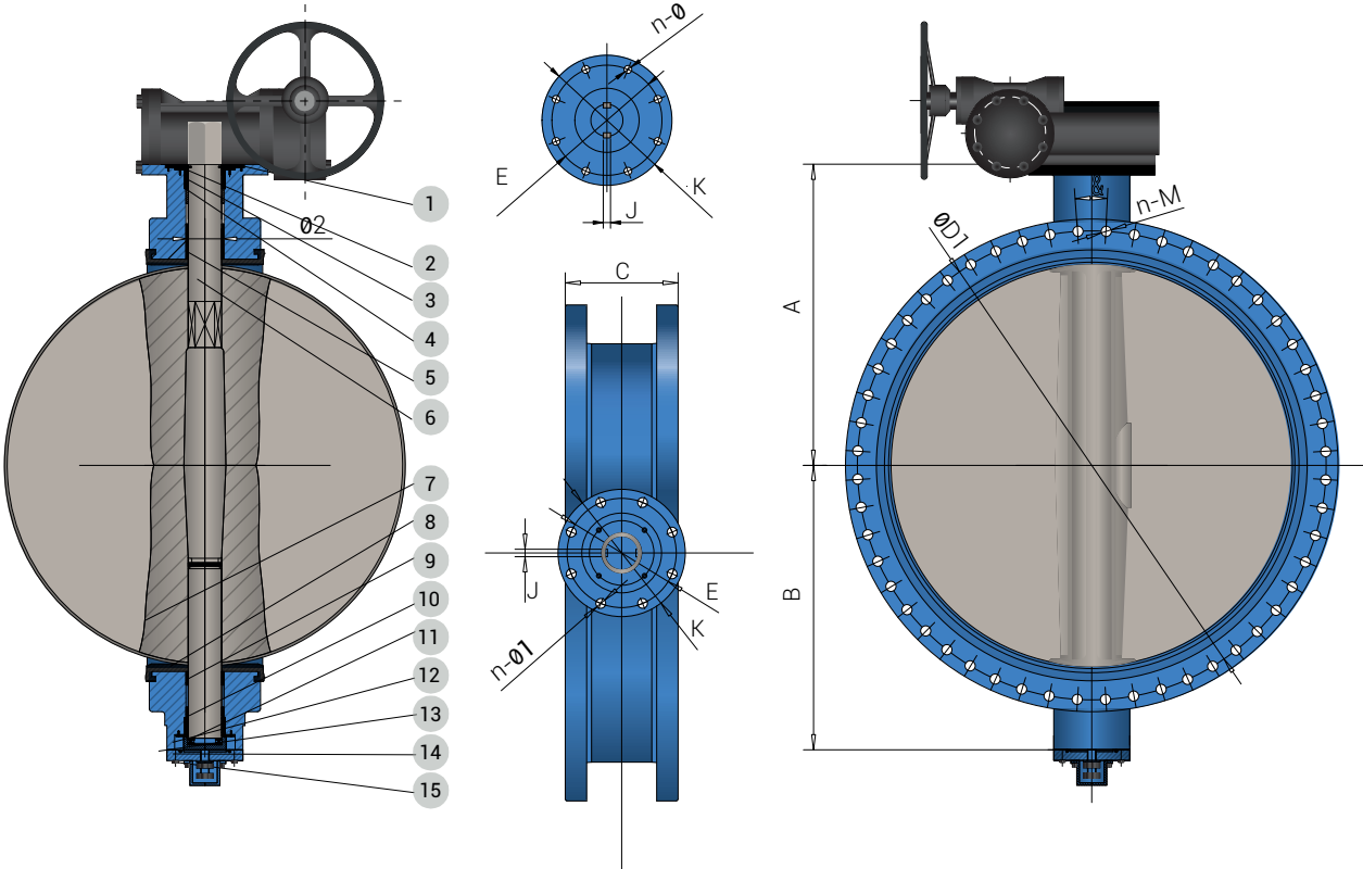
FIG. 4 DN700-1200
