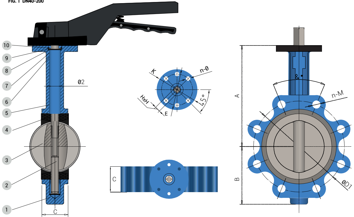
FIG. 1 DN40-200
