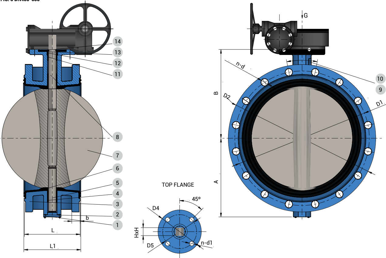
FIG. 3 DN400-600
