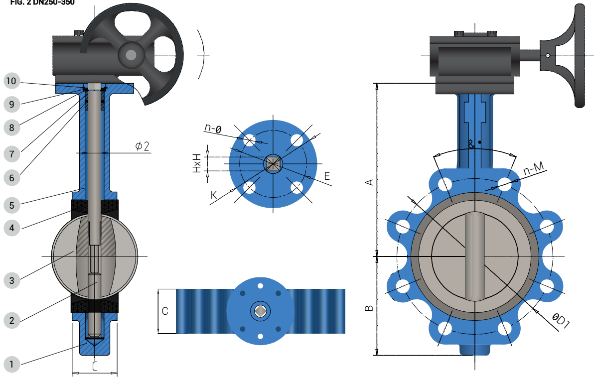
FIG. 2 DN250-350
