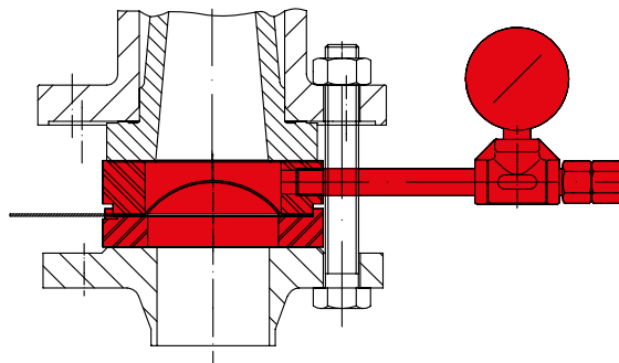
Разрывной диск
