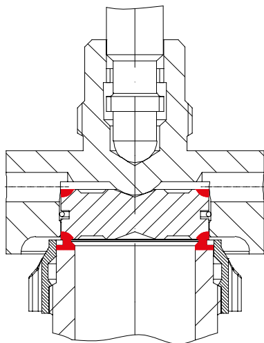
Сопло SA479Gr.316Ti / Стеллит No. 21 Диск затвора SA479Gr.316Ti / Стеллит No. 6
