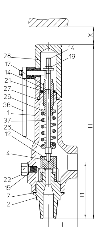
серия ... 966 Рычаг подрыва в закрытом исполнении
