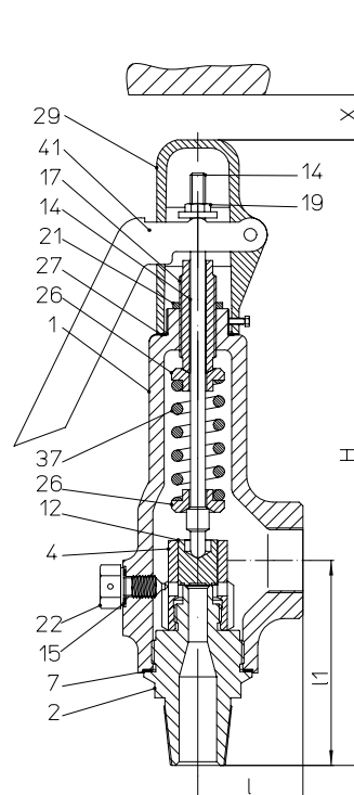
серия ... 969 Рычаг подрыва в открытом исполнении
