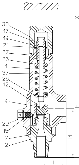
Fig. ... 968 gastight cap
