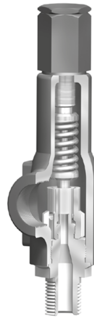
Fig. 968 gastight cap
