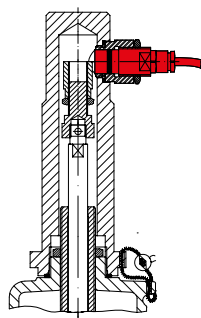
Detector inductivo
