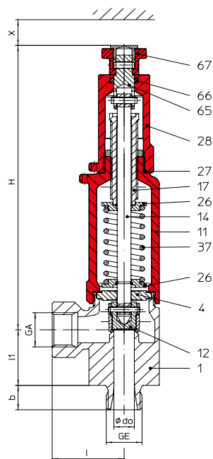
Fig. ... 961 capuchón cerrado
