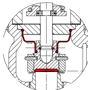
Fig. ... 945 Disco EPDM, inserto blando; fuelle EPDM
