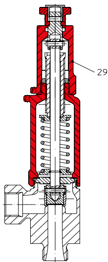
Fig. ... 962 capuchón abierto
