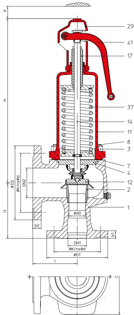
Fig. ... 904 capuchón abierto con palanca, bonete cerrado
