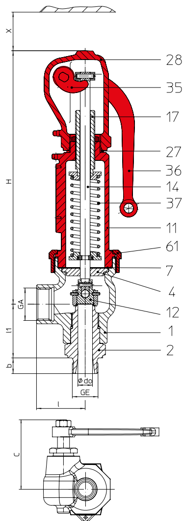
Fig. ... 941 capuchón cerrado con palanca, bonete cerrado
