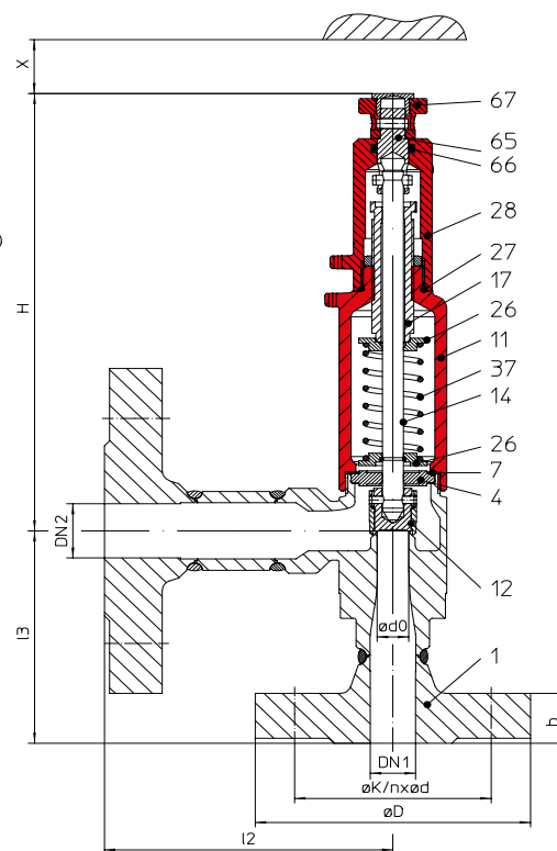
Fig. ... 961 / 962 / 963 opcional con bridas
