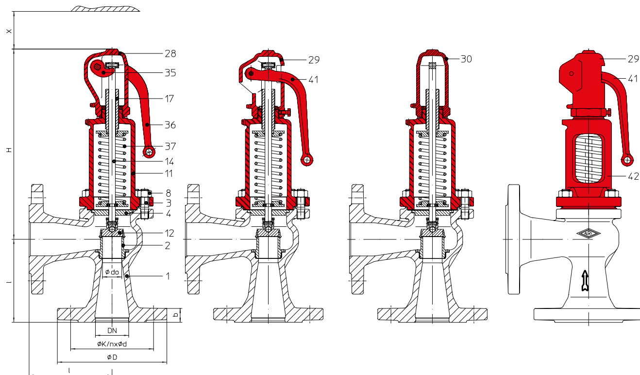
Fig. ... 921 capuchón cerrado con palanca, bonete cerrado
