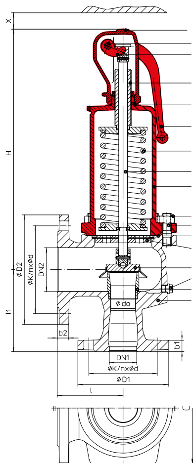
Fig. ... 901 capuchón cerrado con palanca, bonete cerrado
