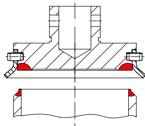
Siège 1.4571 / Stellite n° 21 Clapet 1.4571 / Stellite n° 6 Siège 316Ti / Stellite n° 21 (SAFE-SN ANSI) Clapet 316Ti / Stellite n° 6 (SAFE-SN ANSI) déflecteur de clapet amovible
