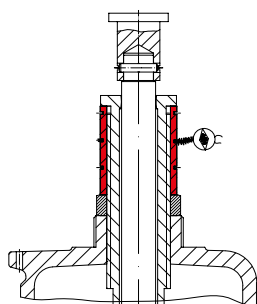
Manchon d'arrêt
