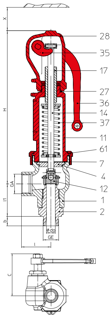
Fig. ... 941 bouchon de levier fermé, chapeau fermé
