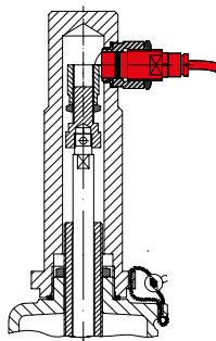
Détecteur de proximité
