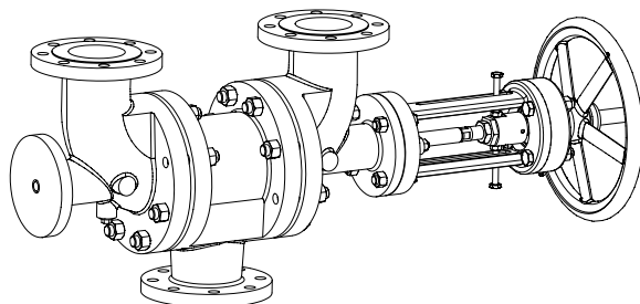
Robinet de jumelage
