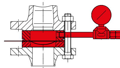
Disque de rupture (Dimensionnement voir page 40.)
