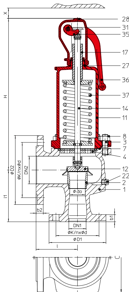
Fig. ... 901 bouchon de levier fermé, chapeau fermé
