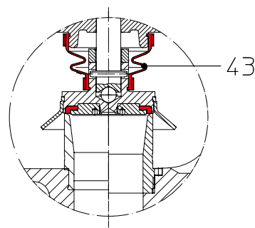
(Construction DN 20-100) (Construction DN125-150) EPDM-disc, soft seal insert; EPDM-bellows
