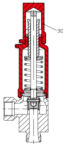
Fig. ... 963 gastight cap
