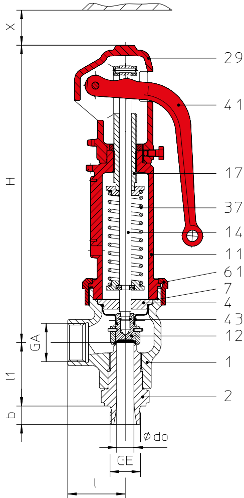
Fig. ....945 otwarty kaptur, zamknięty kołpak
