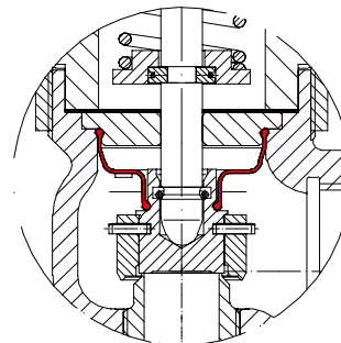
Fig. ....946 Grzybek gniazdo metalowe; mieszek z EPDM
