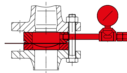
Dysk zrywalny (Projektowanie patrz str. 46.)
