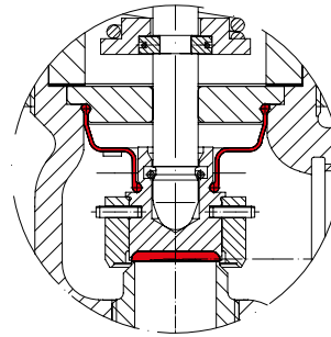
Fig. ....945 Grzybek z EPDM miękki wkład uszcz, mieszek z EPDM
