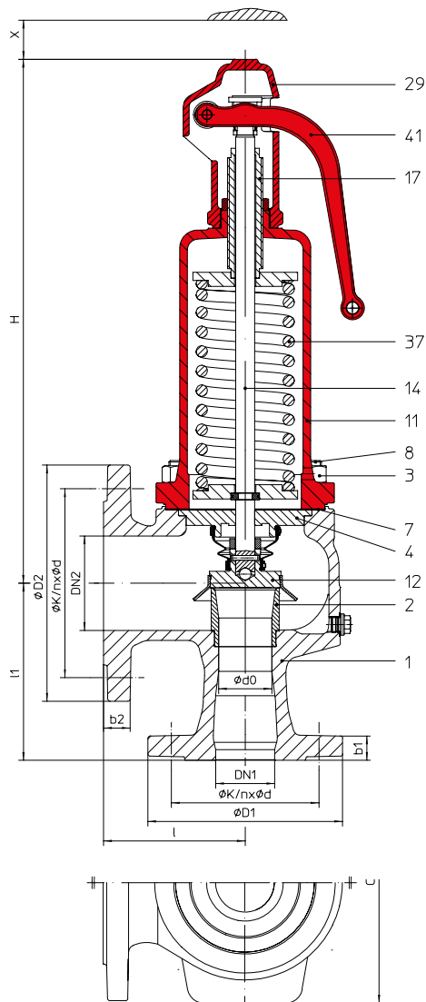
Fig. ... 904 otwarty kaptur, zamknięty kołpak
