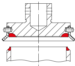
Gniazdo 1.4571 / Stellite No. 21 Grzybek 1.4571 / Stellite No. 6 Gniazdo SA479Gr.316Ti / Stellite No. 21 (SAFE-SN ANSI) Grzybek SA479Gr.316Ti / Stellite No. 6 (SAFE-SN ANSI) Usuwalna pomoc do podnosz.
