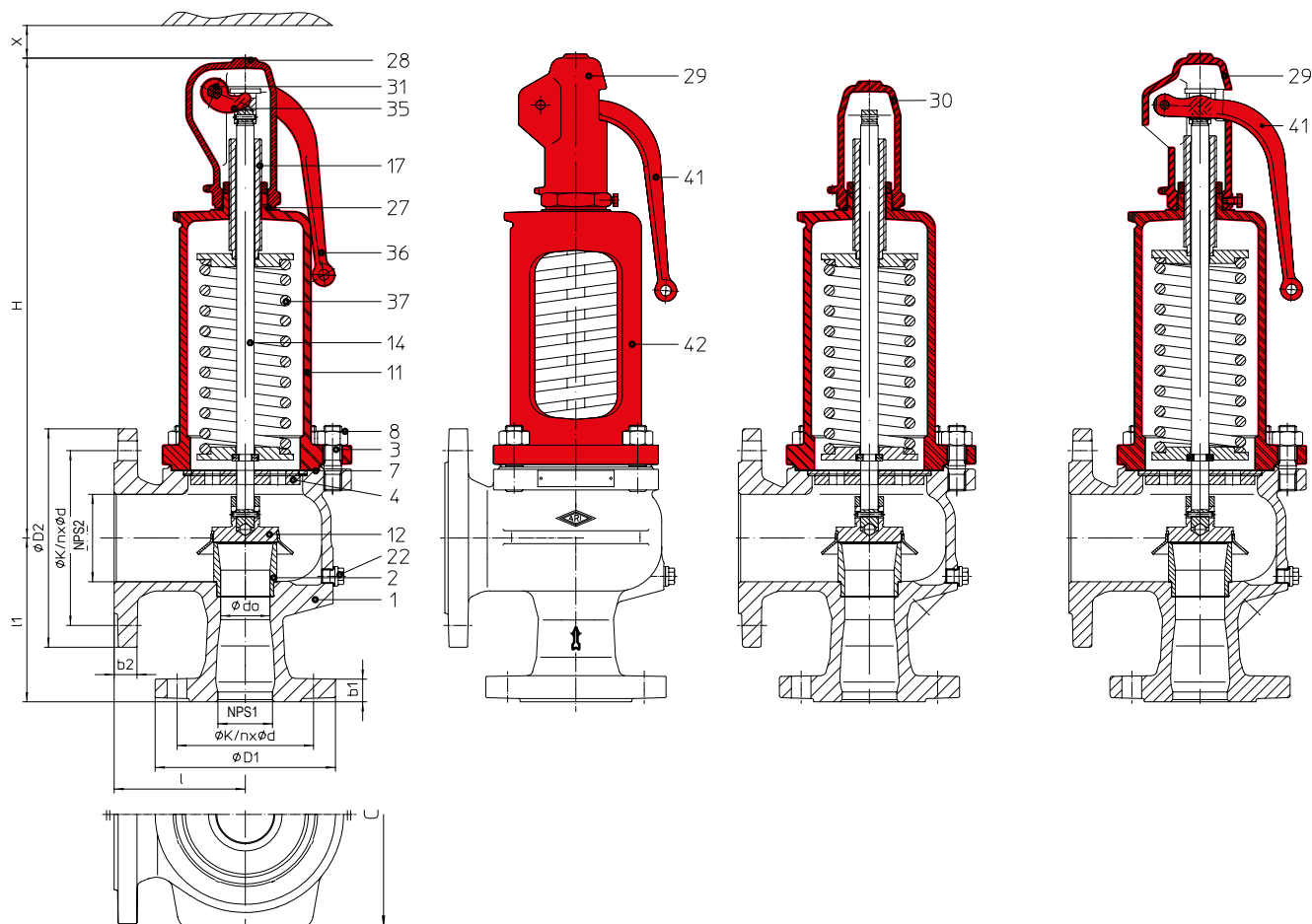
Fig. ... 901 zamknięty kaptur, zamknięty kółpak
