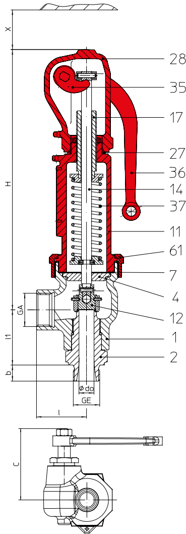
Fig. ... 941 zamknięty kaptur, zamknięty kołpak
