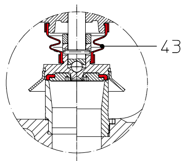
(Wykonanie DN 20-100) (Wykonanie DN125-150) Grzybek z EPDM miękki wkład uszcz, miszek z EPDM
