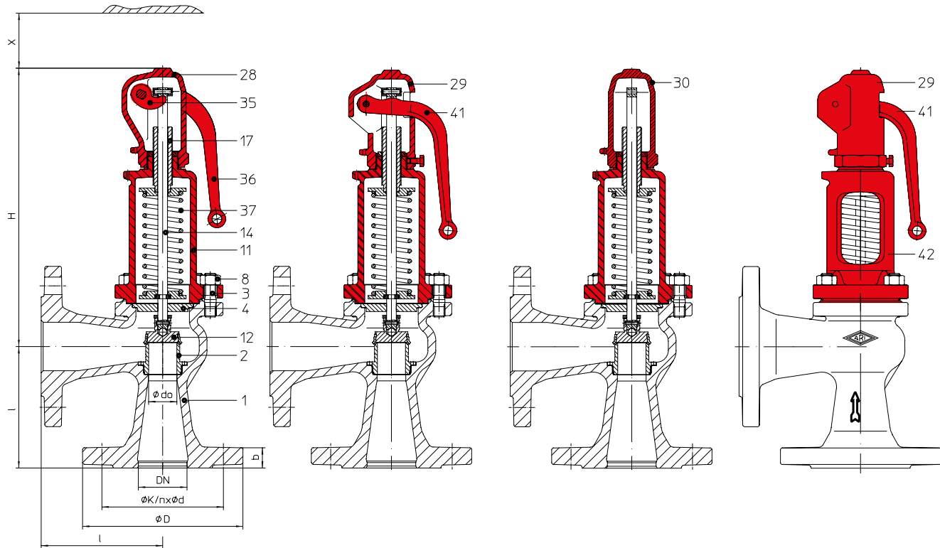
Fig. ... 921 zamknięty kaptur, zamknięty kółpak
