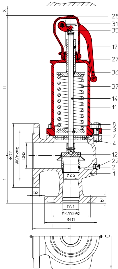
Fig. ... 901 zamknięty kaptur, zamknięty kołpak
