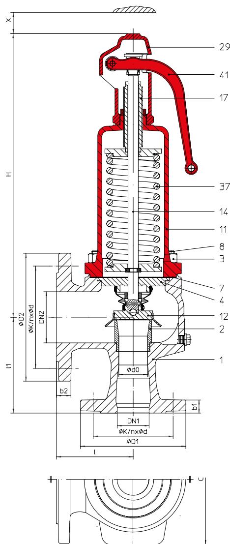
Fig. ... 904 offene Anlüftung, geschlossene Haube
