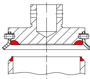
Sitz 1.4571 / Stellite No. 21 Kegel 1.4571 / Stellite No. 6 Sitz 316Ti / Stellite No. 21 (SAFE-SN ANSI) Kegel 316Ti / Stellite No. 6 (SAFE-SN ANSI) lösbare Hubhilfe
