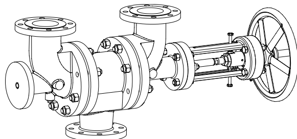
Wechselventil
