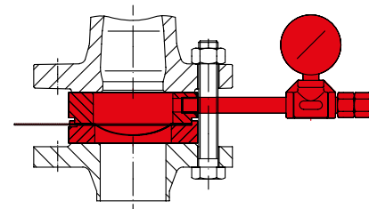
Berstscheibe (Auslegung siehe Seite 46.)
