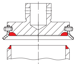
Седло SA479Gr.316Ti / Стеллит No. 21 Затвор SA479Gr.316Ti / стеллит № 6 и съемная оснастка для подъема
