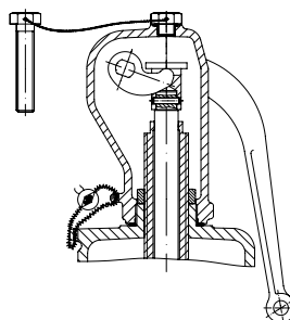
Test gag
