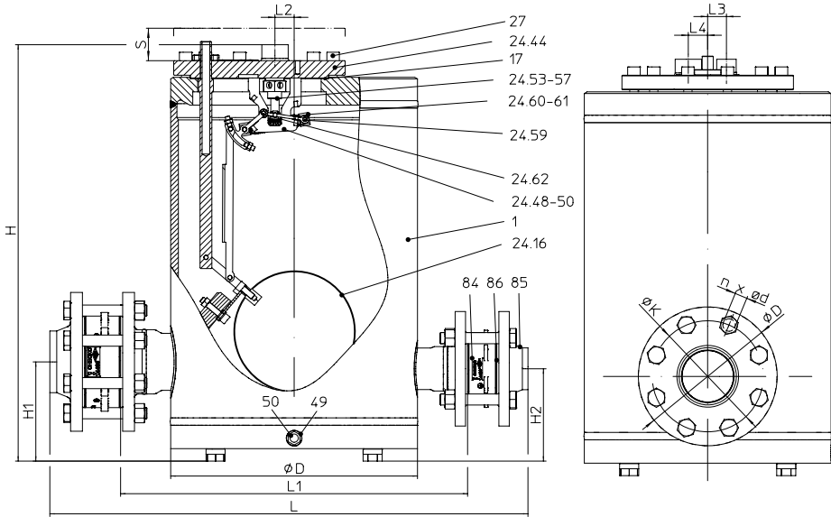
Fig. 691....1 flanşlı
