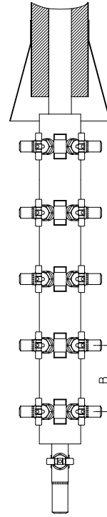
Kondens toplama (B = 160), buhar dağıtımı (B = 120) CODI®S yumuşak salmastralı Fig. 671/672; CODI®B metal körüklü, bakım gerektirmeyen Fig. 675/676
