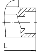
Fig. 640/641....3 soket kaynak boyunlu
