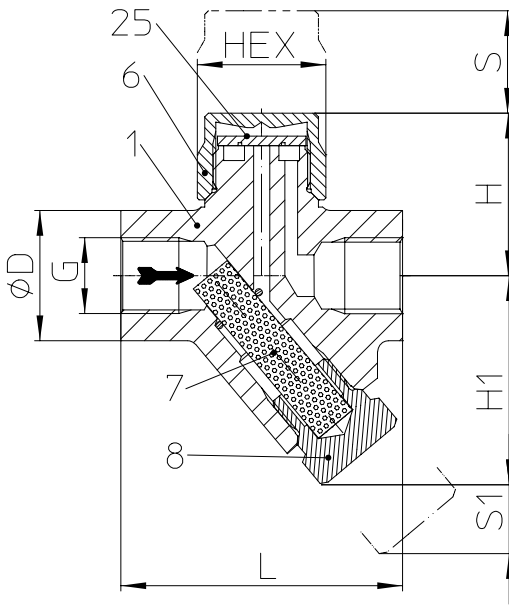
Fig. 641....2 soket dişli
