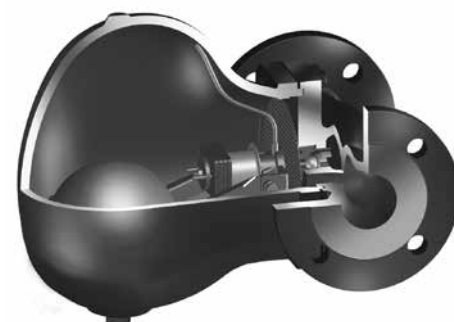
Серия 631....1 горизонтальная установка
