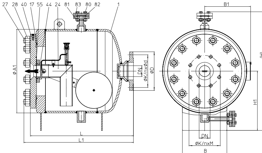
Серия 637....1 Прходное исполнение с фланцами (приток справа)
