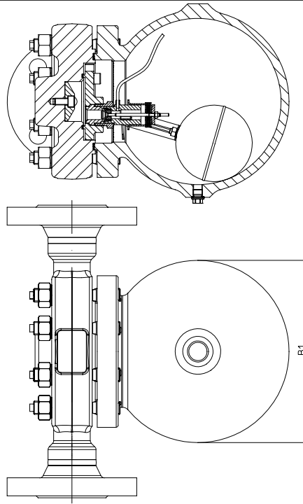
Серия 631....1 Проходное исполнение с фланцами - горизонтальная установка
