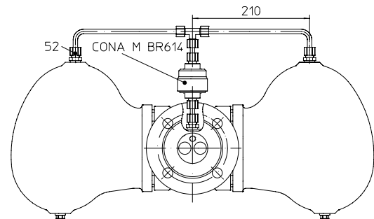
Серия 639....1 с фланцами - горизонтальная установка и внешняя деаэрация
