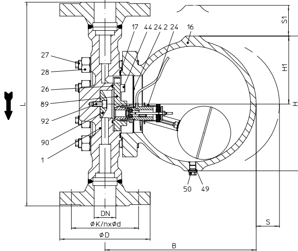
Серия 631....1 Проходное исполнение с фланцами - вертикальная установка
