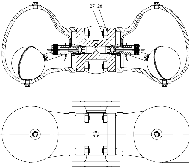
Серия 639....1 с фланцами - горизонтальная установка
