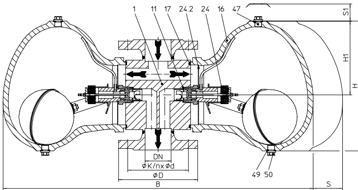
Серия 639....1 с фланцами - вертикальная установка
