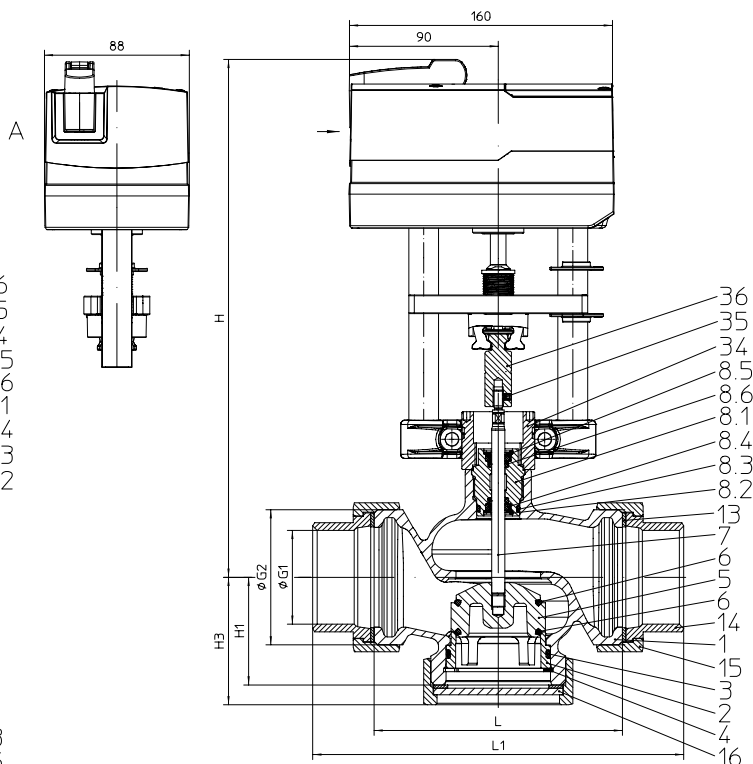
Серия 488 проходной регулирующий
