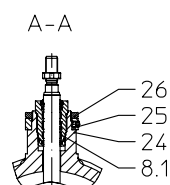
Серия 485 трёхходовой смесительный
