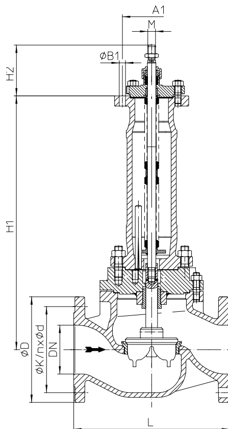
серия 471....90 DN200 / NPS 8" M20 (напр.: DP34-34Tri)
