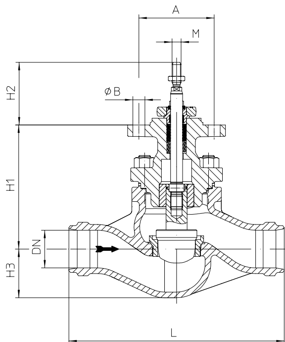
серия 470....4....90 DN25-150 / NPS 1"-6" (напр.: DP32-34; PREMIO 2,2-25kN; AUMA 07.2-10.2)
