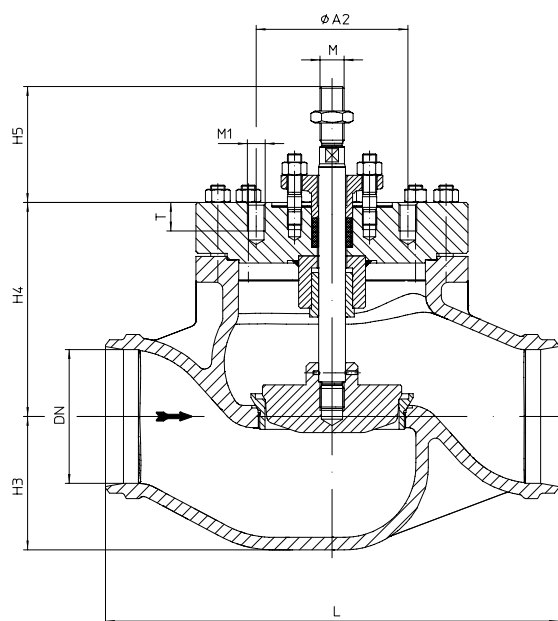
серия 470...4...90 DN150 / NPS 6" (напр.: DP35; AUMA 14.2-14.6)
