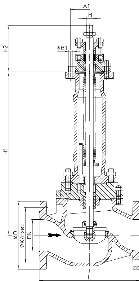
серия 471....90 DN150 / NPS 6" (напр.: DP34T-35; AUMA 14.2)
