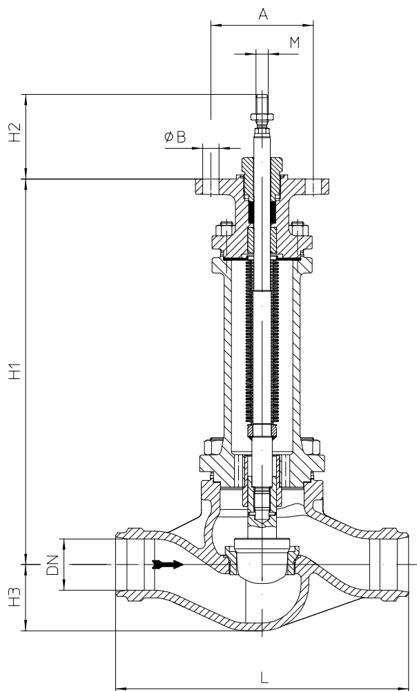
серия 471....4....90 DN25-150 / NPS 1"-6" (напр.: DP32-34; PREMIO 2,2-25kN; AUMA 07.2-10.2)
