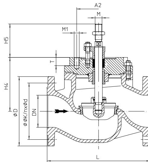
серия 470....90 DN150-200 / NPS 6"-8" (напр.: DP35; AUMA 14.2-14.6)
