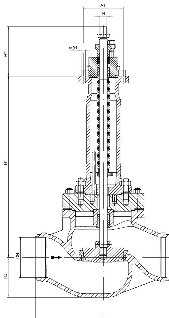
серия 471...4...90 DN150 / NPS 6" (напр.: DP34T-35; AUMA 14.2)
