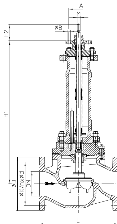
серия 471....90 DN200 / NPS 8" M16 (напр.: PREMIO 5-25kN, AUMA 07.6-10.2)
