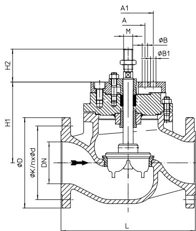
серия 470....90 DN200 / NPS 8" (напр.: DP34, PREMIO 5-25kN)
