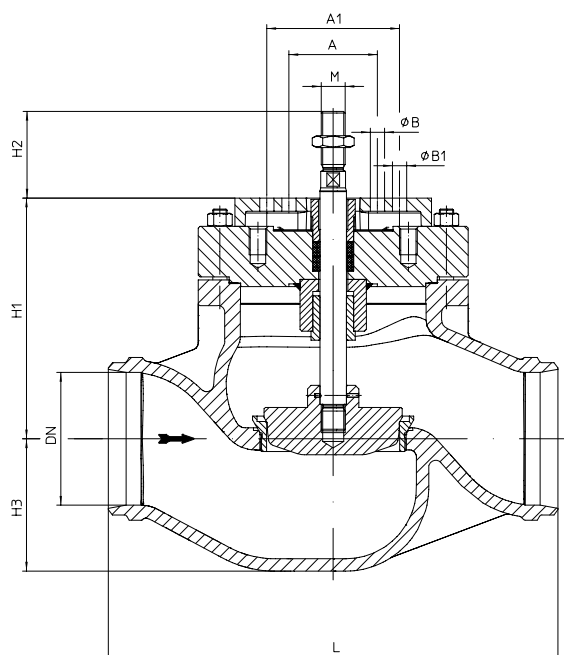
серия 470...4...90 DN150 / NPS 6" (напр.: DP34T-34Tri)
