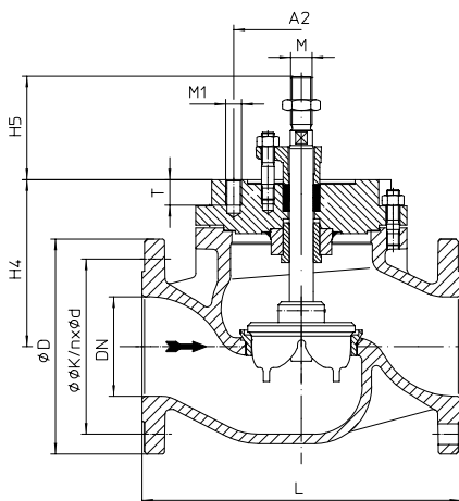
серия 470....90 DN200 / NPS 8" (напр.: AUMA 07.6-10.2)
