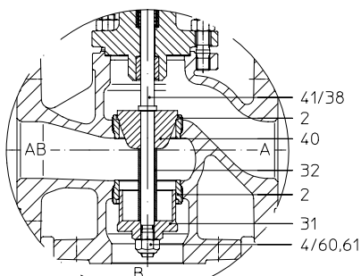
Плунжер разделительный начиная с DN 40
