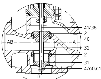
Плунжер раздельный начиная с DN 40
