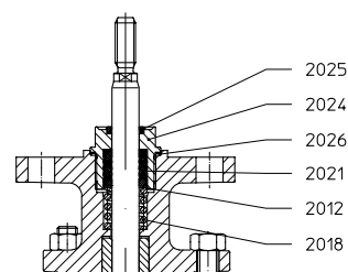
III. Сильфон нержавеющей с шевронными манжетами PTFE
