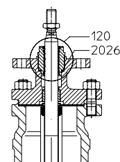
III. Сильфон нержавеющей с уплотнением EPDM
