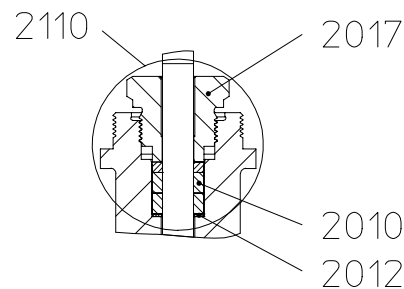
III. Сильфон нержавеющей с сальником графитовым
