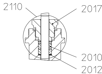
III. Soufflet inox et garniture d'étanchéité en graphite pur
