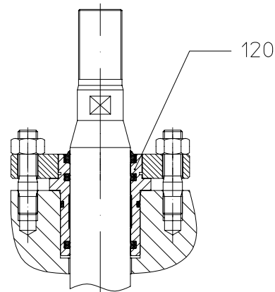
I. Уплотнение EPDM
