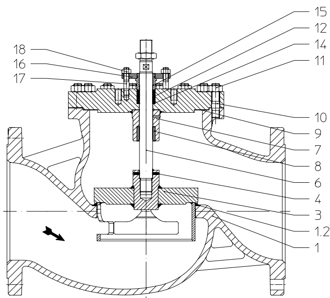
II. Сальниковое уплотнение PTFE- / Сальниковое уплотнение графит
