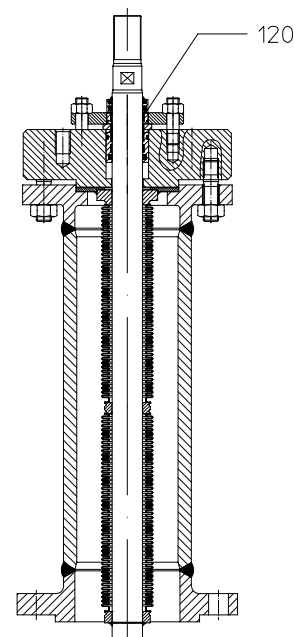
III. Сифон нержавеющий с уплотнением EPDM
