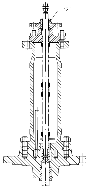
III. Сифон нержавеющий с уплотнением EPDM
