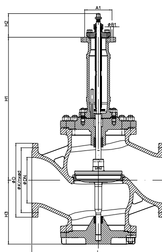
Серия 462 DN200-250 M20 (напр.: DP34-34Tri)
