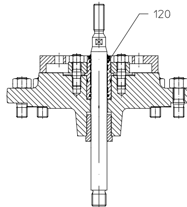
I. Уплотнение EPDM
