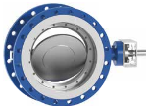
Fig. 122 - ARI-ZEDOX® Doppelflansch
