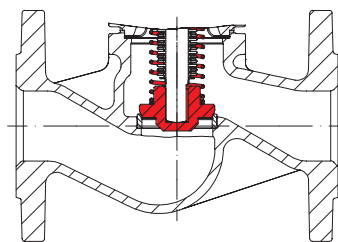
Otturatore con funzione di ritegno con sede a spigolo e molla di richiamo Pressione di taratura 0,1 bar
