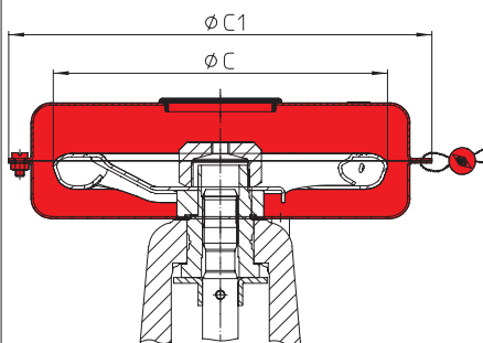
Valvola con cappuccio piombato acc. to DIN EN 12828 (protezione antimanomissione del volante)
