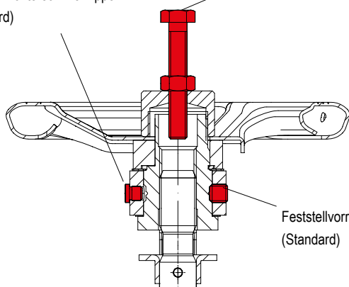
Flacher Trichterschmiernippel / Feststellvorrichtung / Hubbegrenzung
