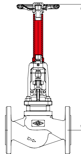
Spindelverlängerung (Höhe bei Bestellung angeben!)
