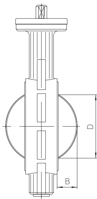
Saillie du robinet par rapport à la longueur face à face
