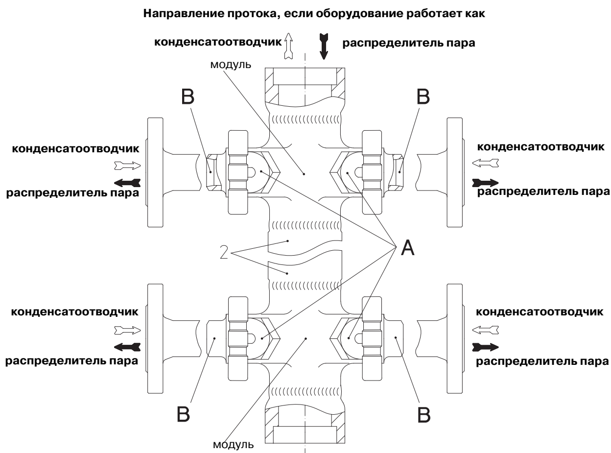
Крепеж для сборника конденсата / распределителя пара
