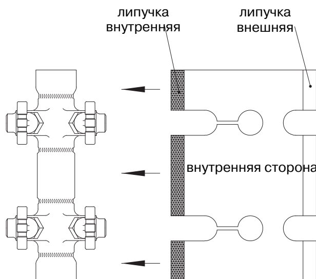
Рис. 6: базовая изоляция
