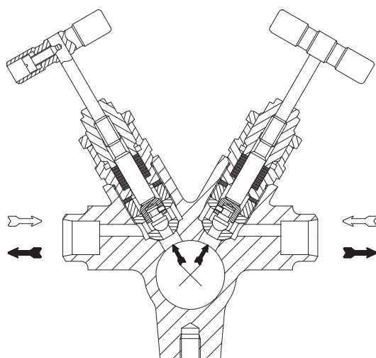
CODI® S avec étanchéité à presse-étoupe PN40 / PN63 / Class 150 / Class 300
