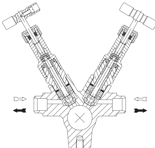
CODI® B avec étanchéité à soufflet PN40 / PN63 / Class 150 / Class 300
