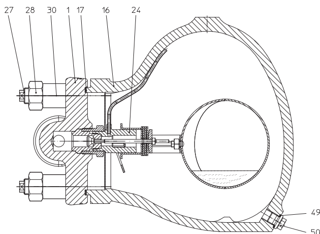
obr. 7a: CONA ® S - BR631 PN63
