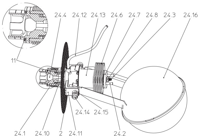
obr. 7b: Sestava plovákového regulátoru
