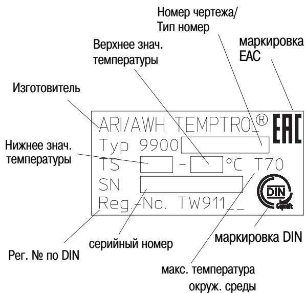
Рис. 2: Клапан
