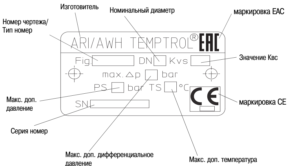
Рис. 2: Клапан
