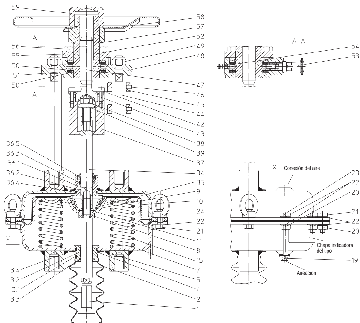
Fig. 4: DP30 / DP32 con reajuste manual de emergencia "Vástago en posición retraída"
