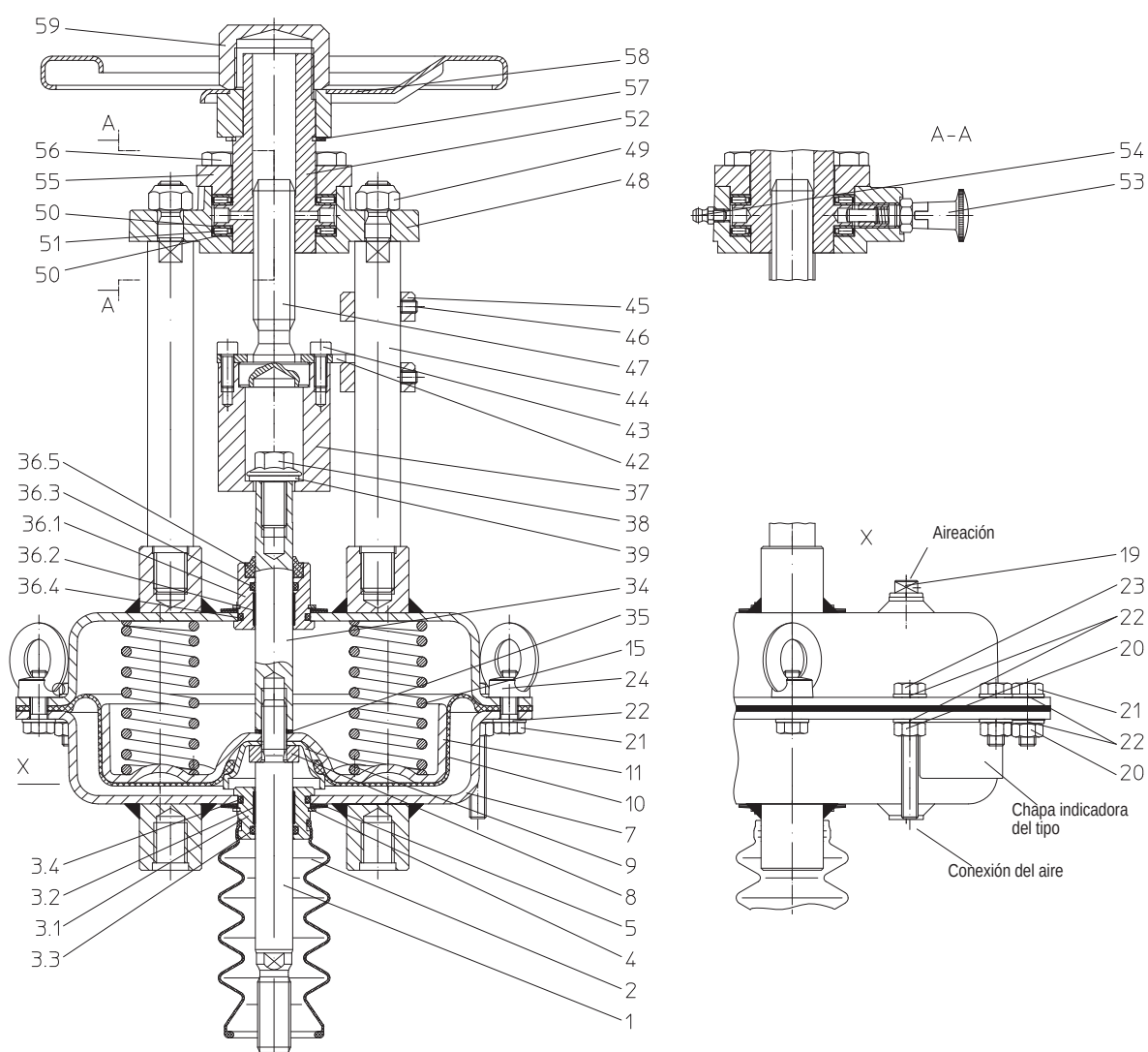
Fig. 2: DP30 / DP32 con reajuste manual de emergencia "Vástago en posición extendida"
