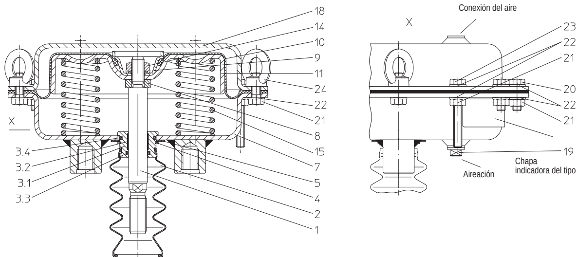
Fig. 3: DP30 / DP32 "Vástago en posición retraída"
