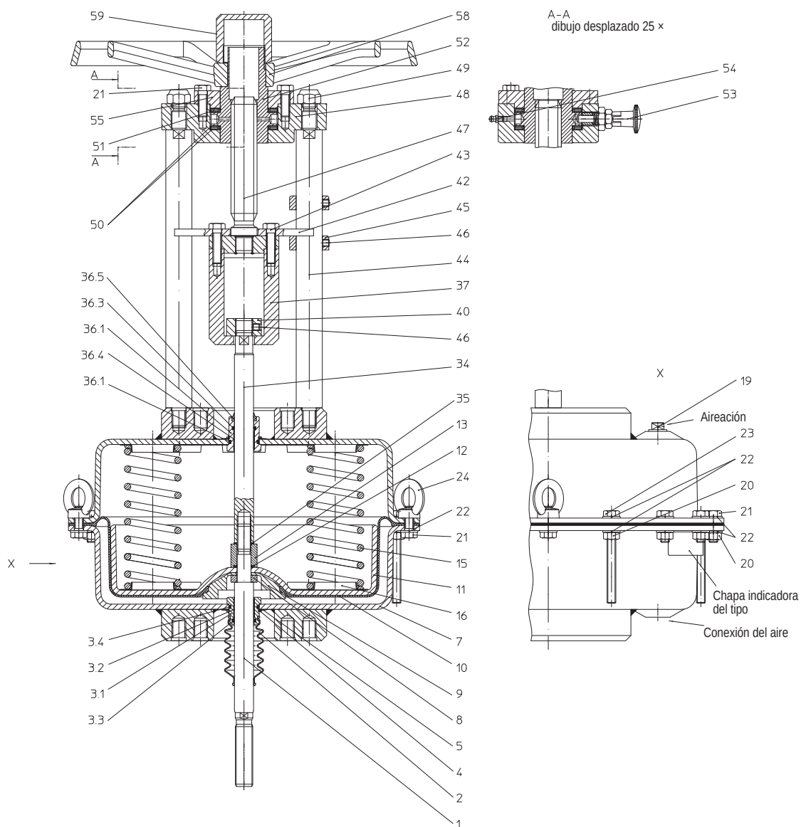
Fig. 10: DP34 con reajuste manual de emergencia "Vástago en posición extendida"
