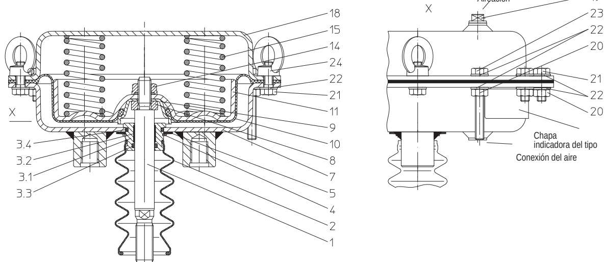
Fig. 1: DP30 / DP32 "Vástago en posición extendida"
