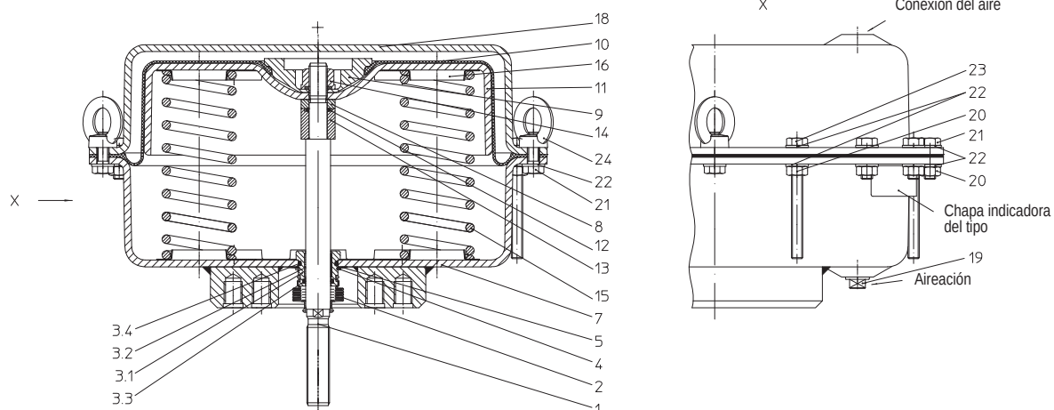
Fig. 11: DP34 "Vástago en posición retirada"
