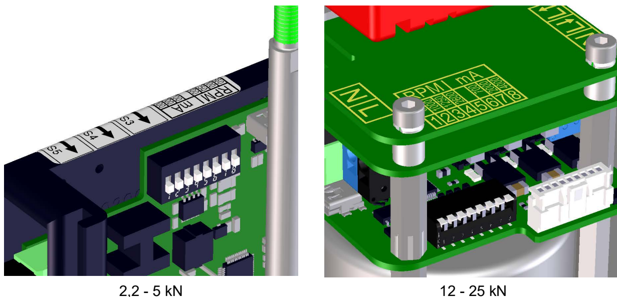
Bild 5: DIP-Schalter auf der Motorsteuerplatine
