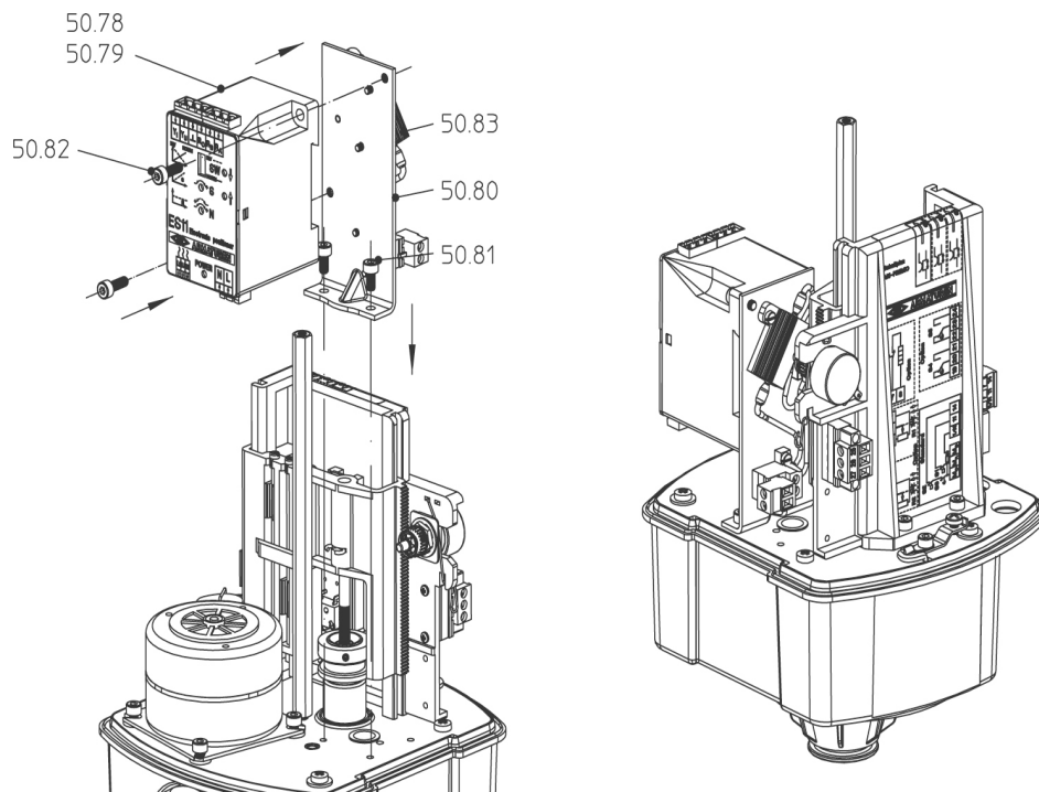
Bild 15: Einbau RI21 / ES11 / Heizung ARI-PREMIO® 2,2 - 5 kN
