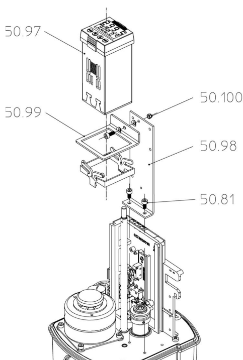
Bild 18: Einbau dTRON 316 ARI-PREMIO® 2,2 - 5 kN
