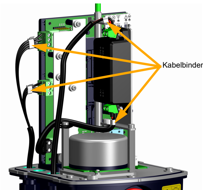
Bild 6: Einzeladern mit Kabelbinder
