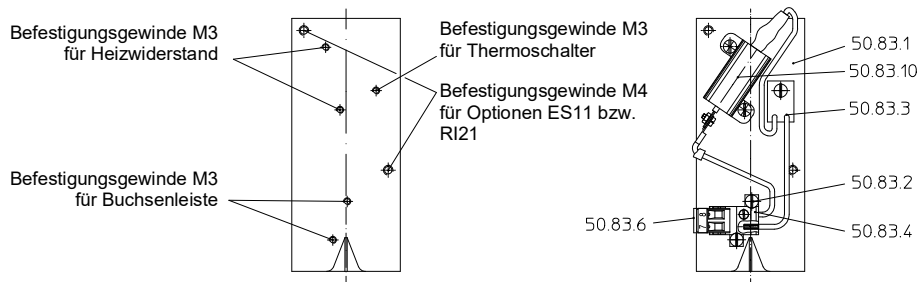
Bild 14: Einbau Heizung ARI-PREMIO® 2,2-15 kN
