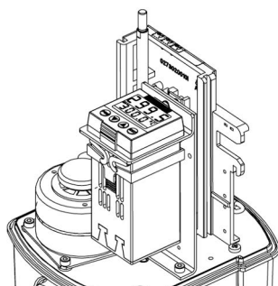
Bild 18: Einbau dTRON 316 ARI-PREMIO® 2,2 - 5 kN
