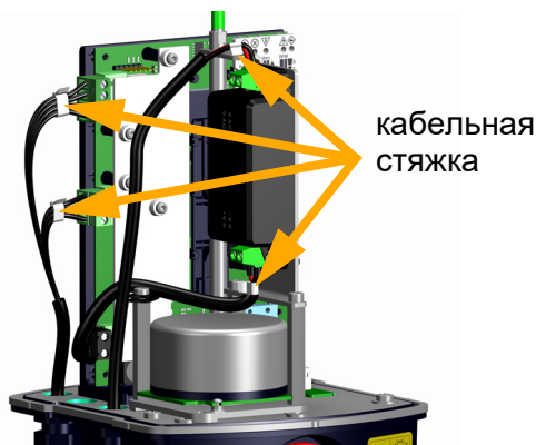
рис. 2: Отдельные жилы в кабельной стяжке
