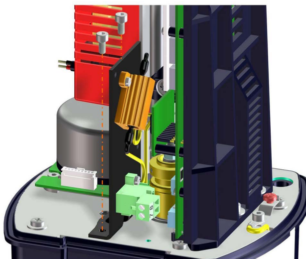
рис. 11: Монтаж обогрева ARI-PREMIO®-Plus 2G 2,2 - 25 кН
