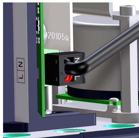
Bild 14: Einbau und Anschluss Netzteil ARI-PREMIO®-Plus 2G 9 kN mit Sicherheitsfunktion und ARI-PREMIO®-Plus 2G 25 kN
