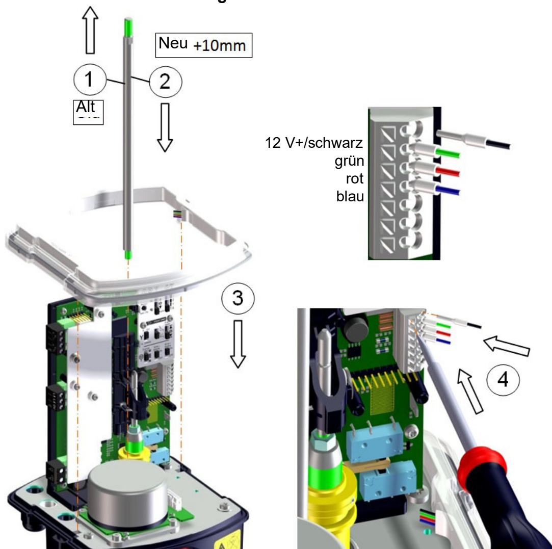
Bild 15: Einbau und Anschluss der LED-Statusanzeige
