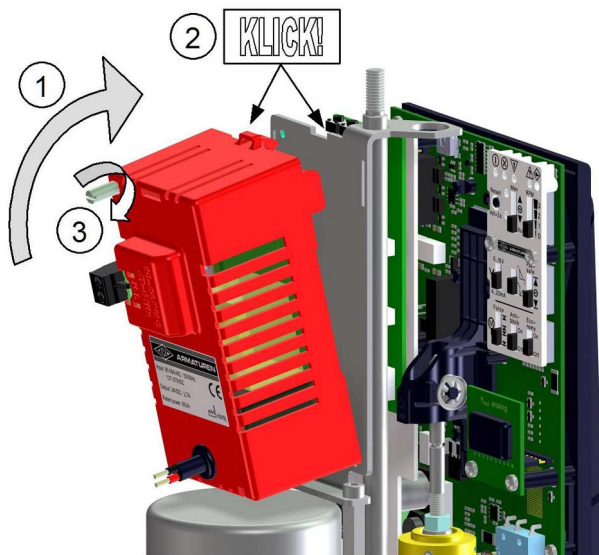
Bild 14: Einbau und Anschluss Netzteil ARI-PREMIO®-Plus 2G 9 kN mit Sicherheitsfunktion und ARI-PREMIO®-Plus 2G 25 kN
