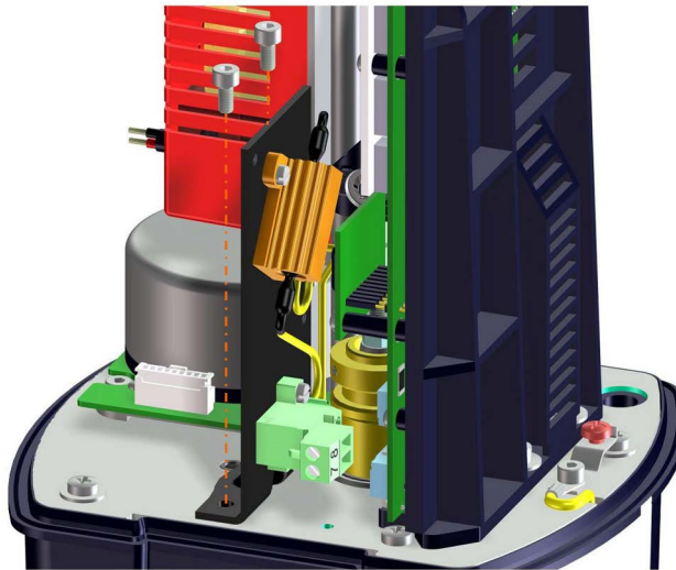
Bild 11: Einbau Heizung ARI-PREMIO -Plus 2G 2,2 - 25 kN
