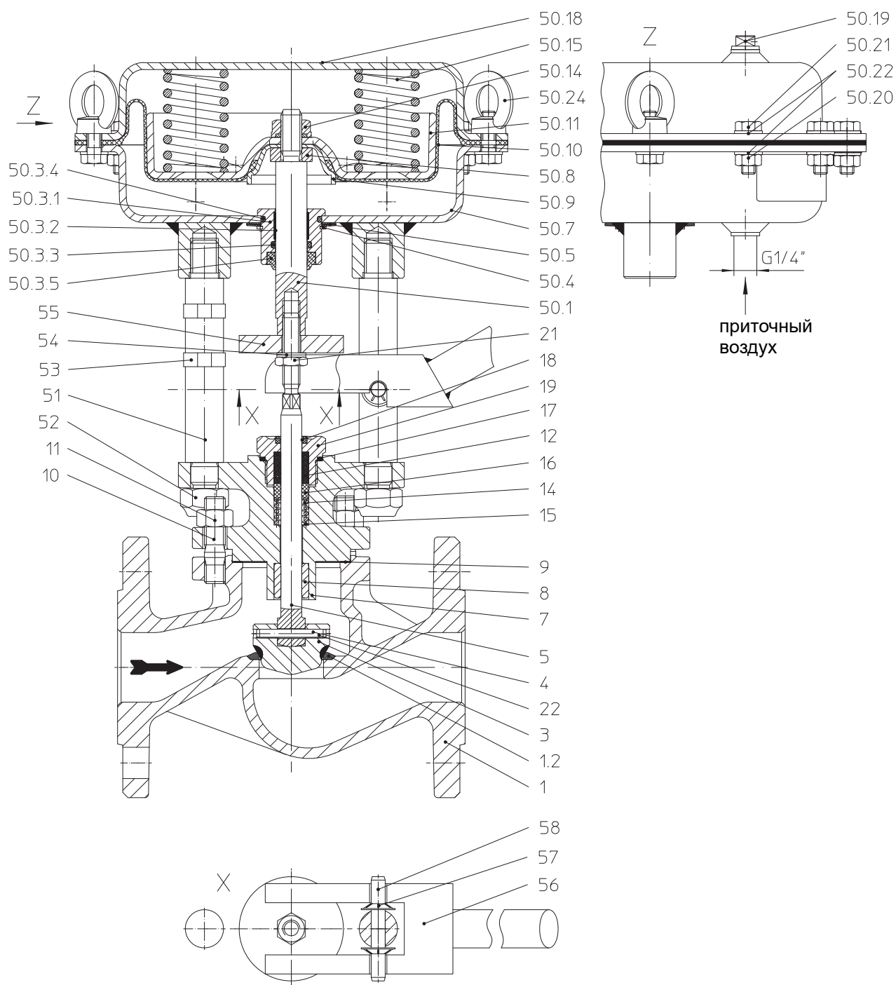
Рис. 2: BR 415 DN 40, 50
