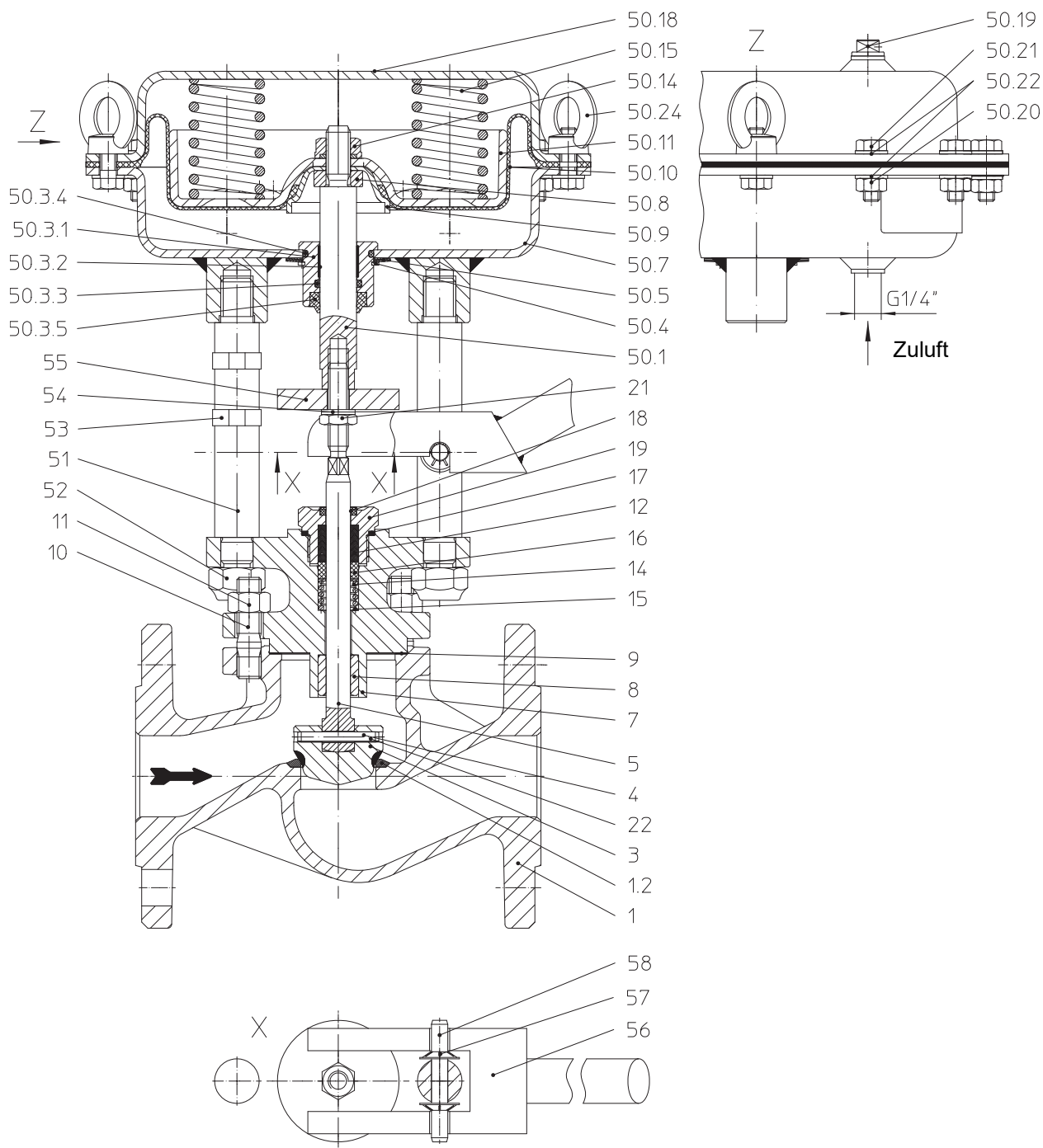
Bild 2: BR 415 DN 40, 50
