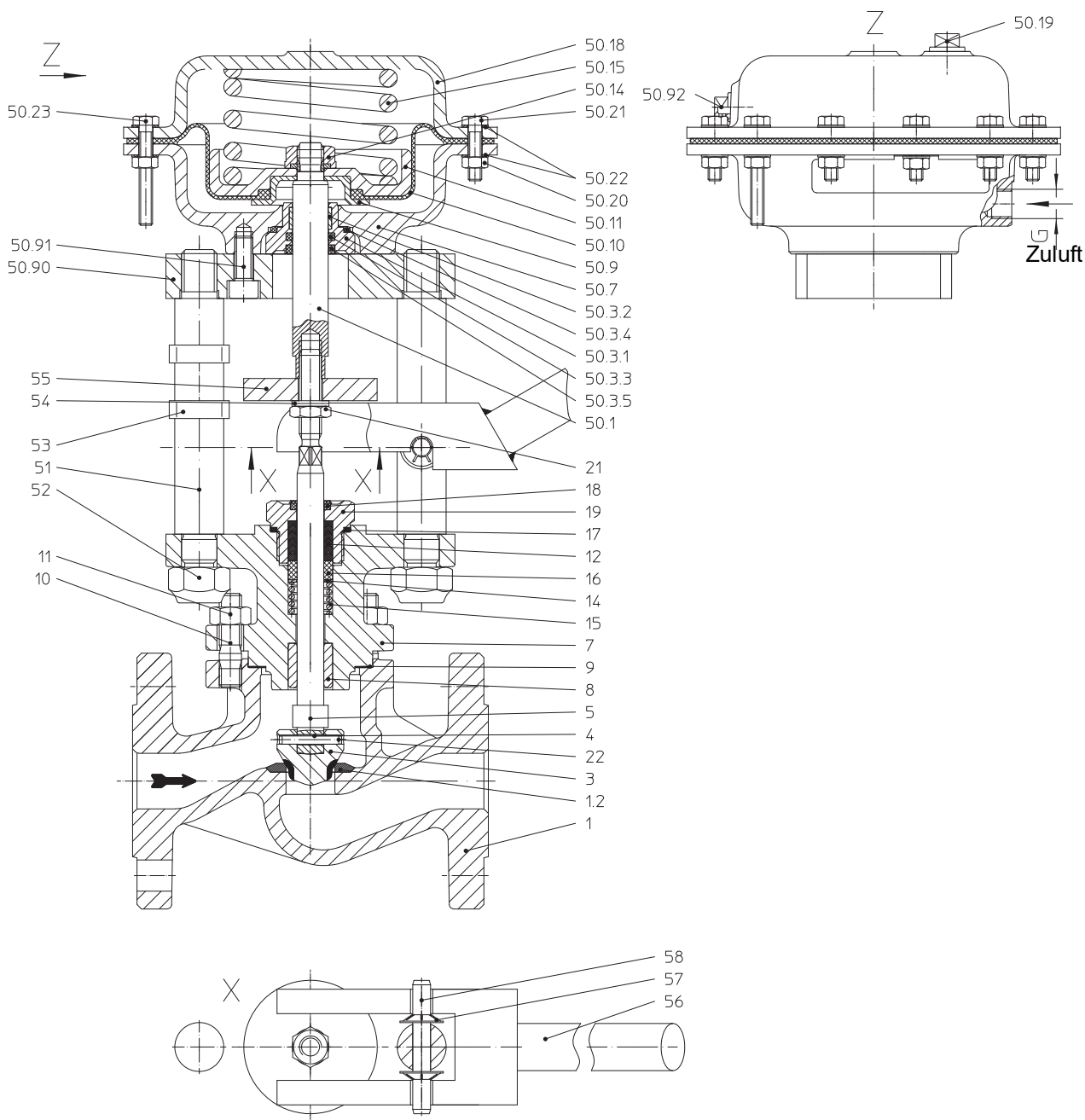
Bild 1: BR 415 DN 25, 32
