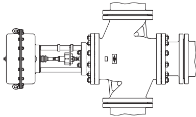
Bild 4: Rohrleitung senkrecht
