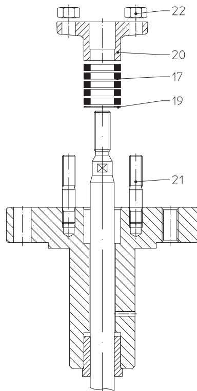
Bild 7: Stopfbuchspackung
