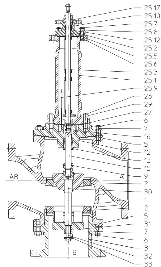
Рис. 4: BR 463
