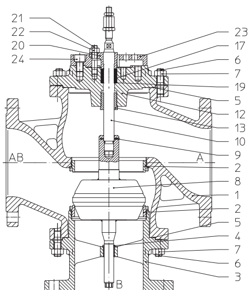
Рис. 1: BR 423
