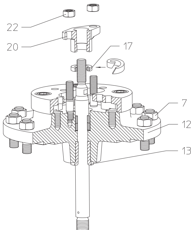
Рис. 8: сальниковая набивка
