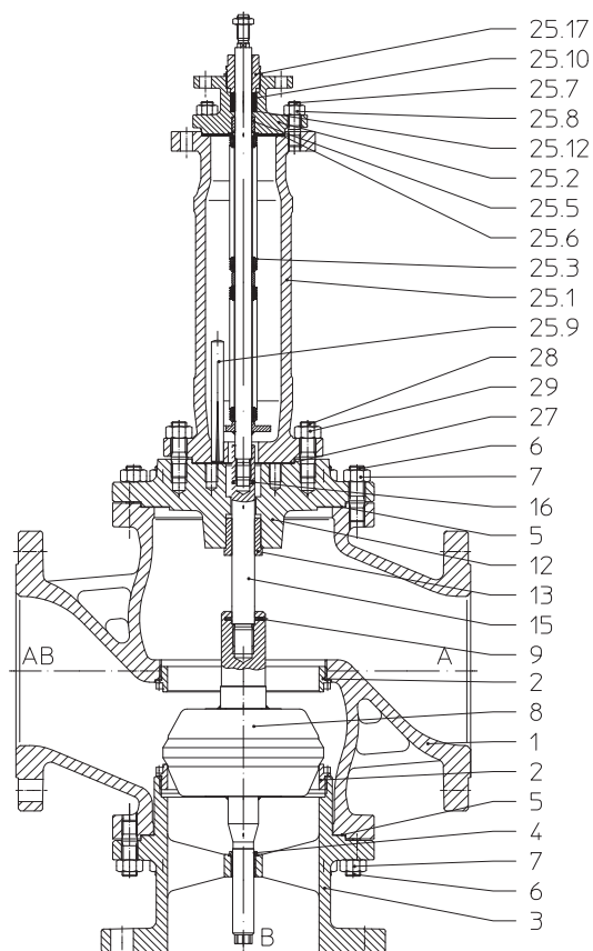
Рис. 2: BR 463
