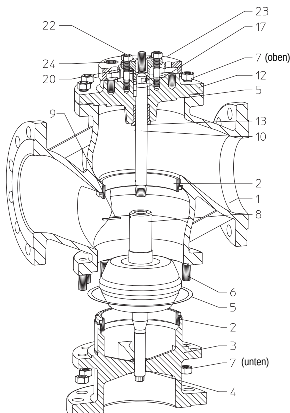
Rys. 12: BR423 z grzybkiem stożkowym mieszającym
