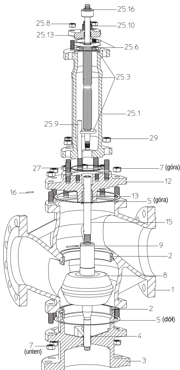
Rys. 10: BR 463 z grzybkiem stożkowym mieszającym
