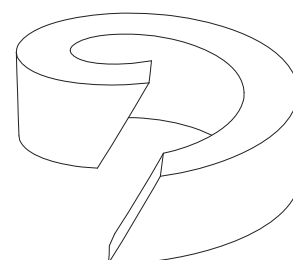
Rys. 9: Dzielony pierścień uszczelniający
