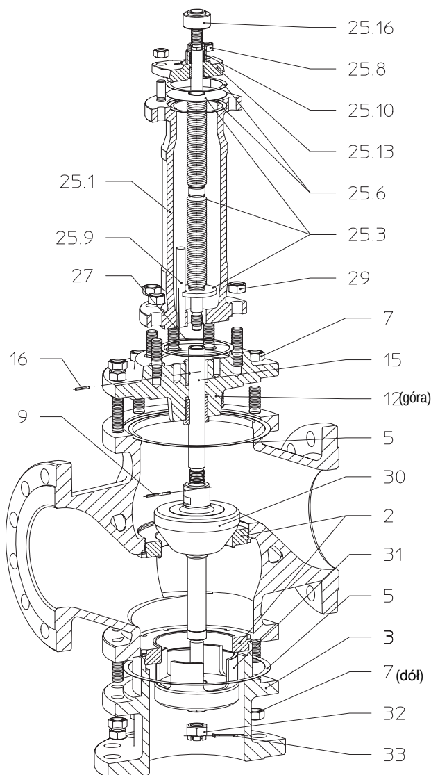
Rys. 11: BR 463 ze stożkiem rozdzielającym
