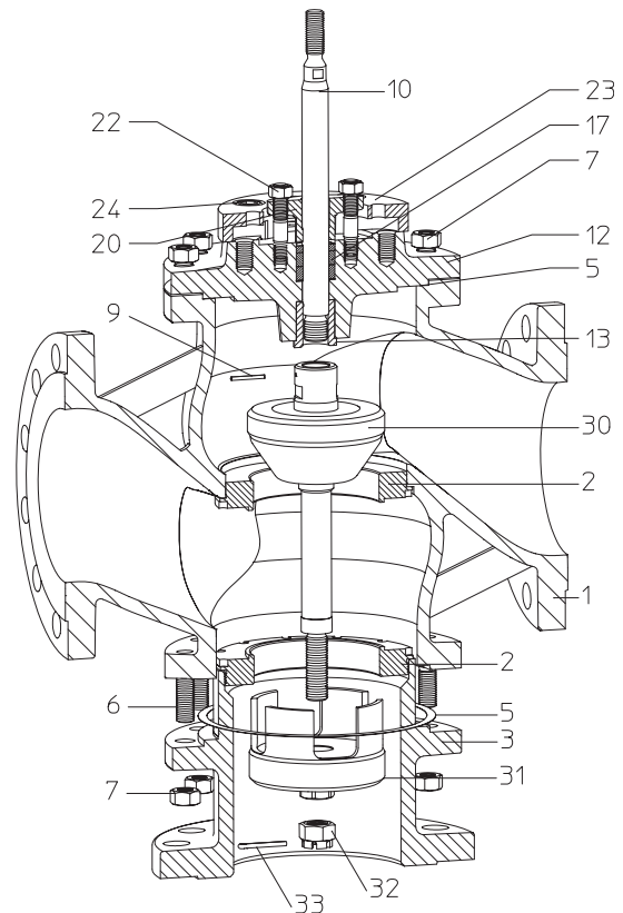
Bild 14: BR423 mit Verteilkegel
