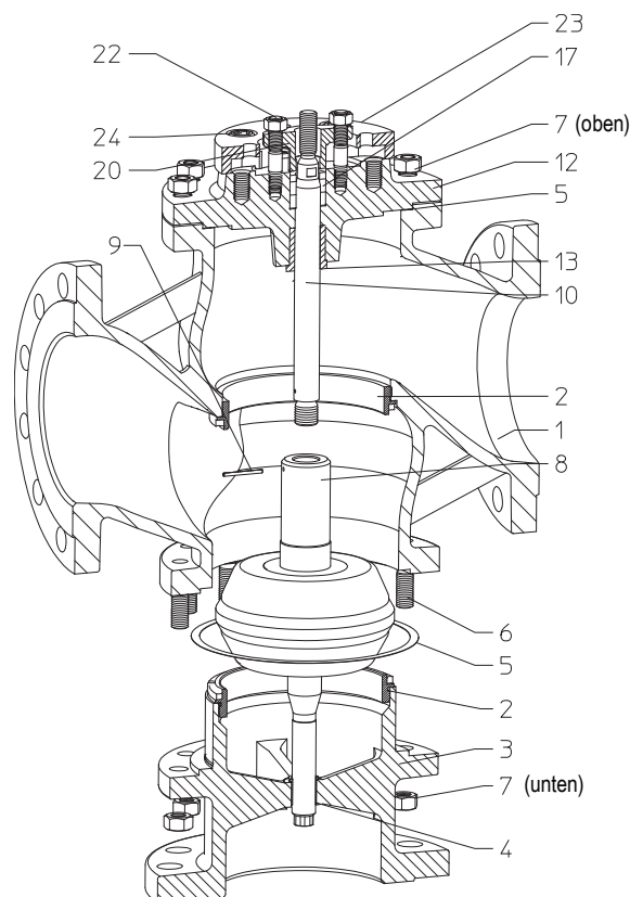
Bild 13: BR423 mit Mischkegel
