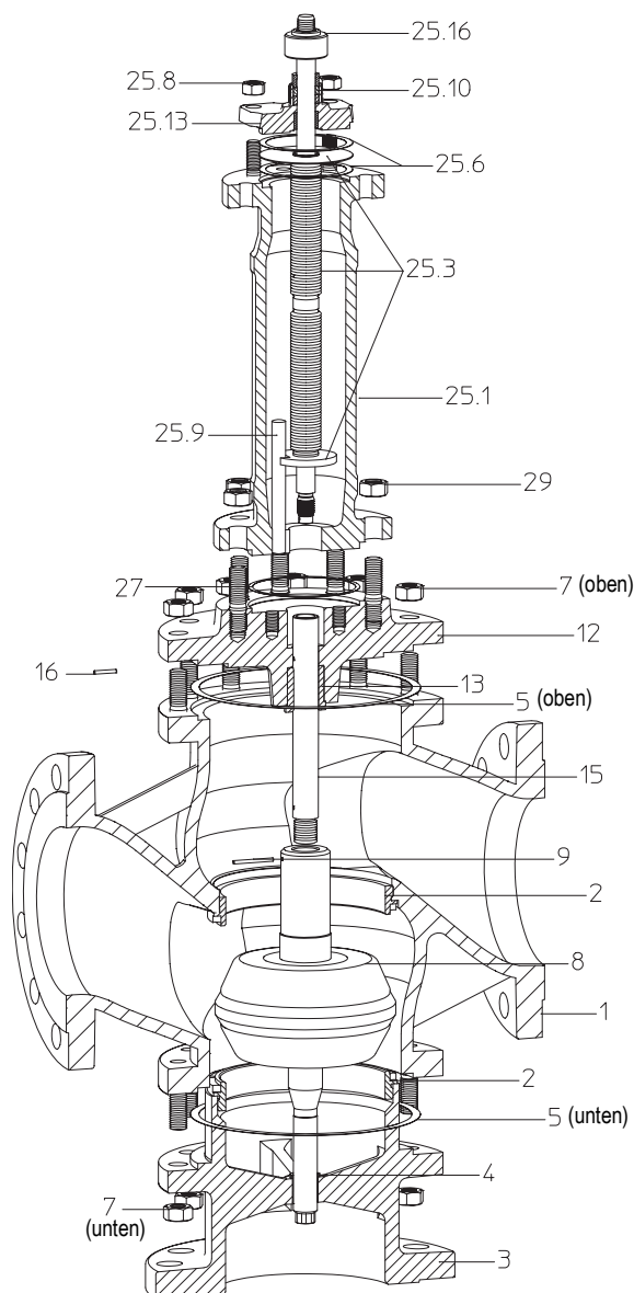
Bild 11: BR 463 mit Mischkegel
