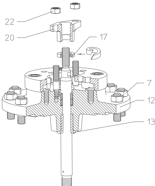
Bild 8: Stopfbuchspackung
