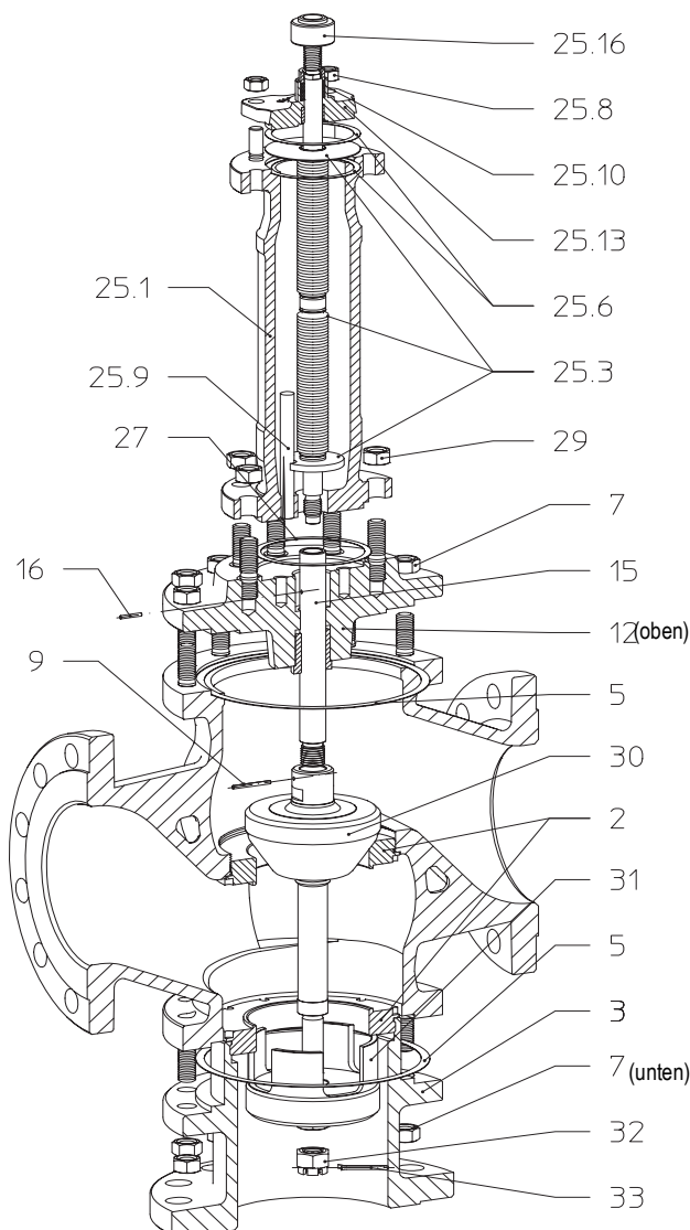
Bild 12: BR 463 mit Verteilkegel
