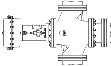
Bild 6: Rohrleitung senkrecht
