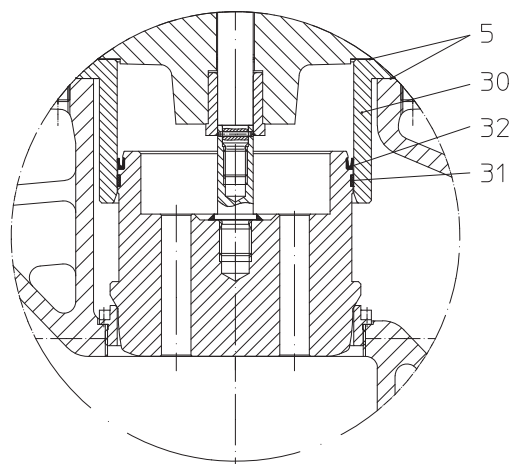
Рис. 11: затвор для понижения давления
