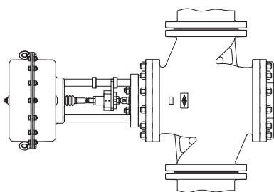
Рис. 5: вертикальный трубопровод
