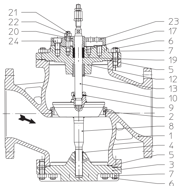
Рис. 1: BR 422
