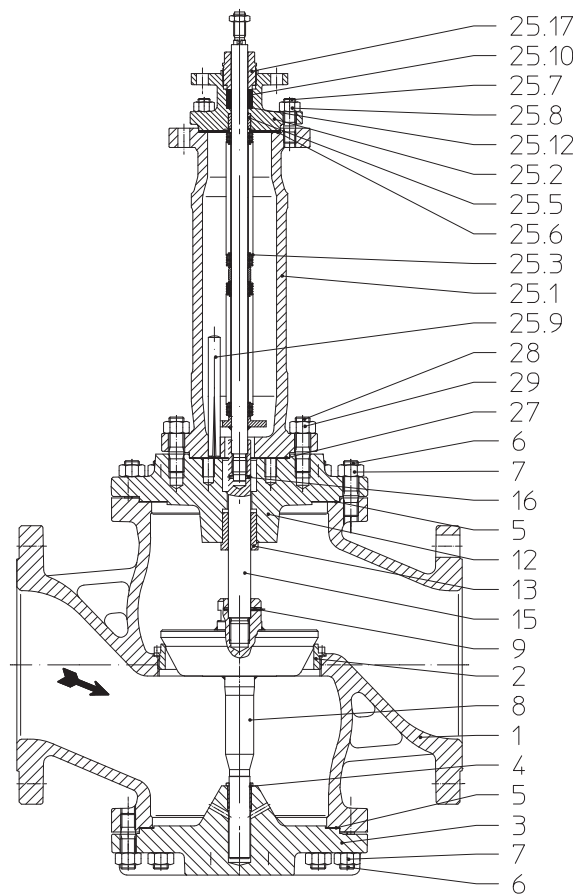
Рис. 2: BR 462
