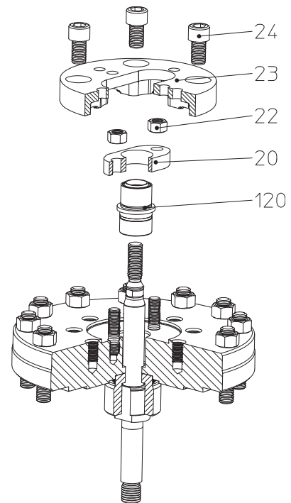
Bild 9: EPDM Abdichtung
