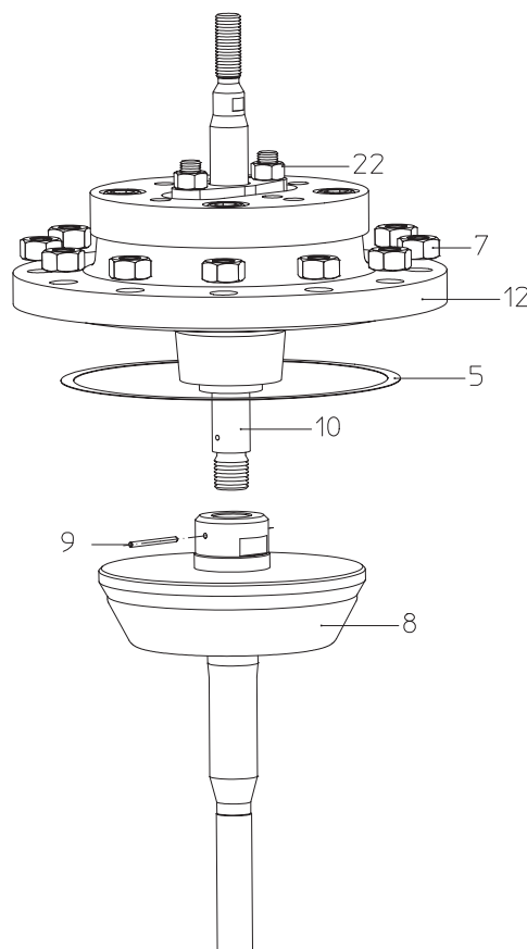
Bild 11: BR 422
