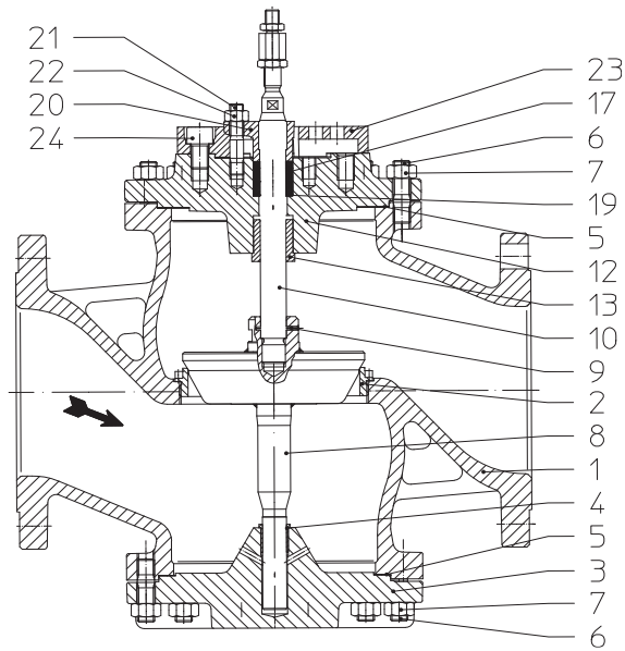
Bild 1: BR 422
