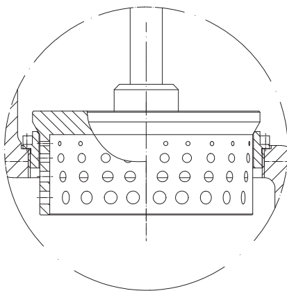
Bild 3: Lochkegel
