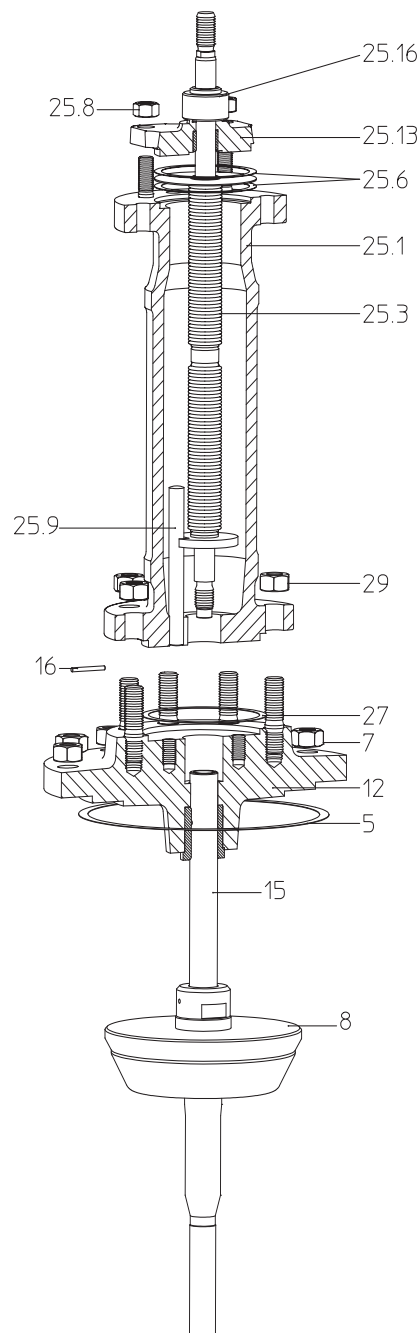
Bild 10: BR 462
