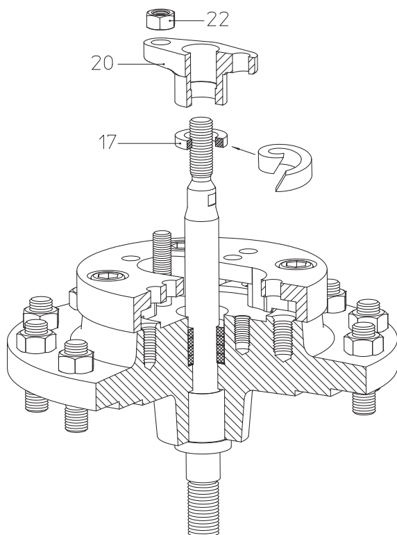
Bild 7: Stopfbuchspackung
