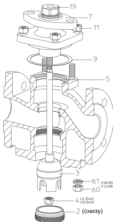
Рис. 20: BR450 DN15-150 со смесительным затвором
