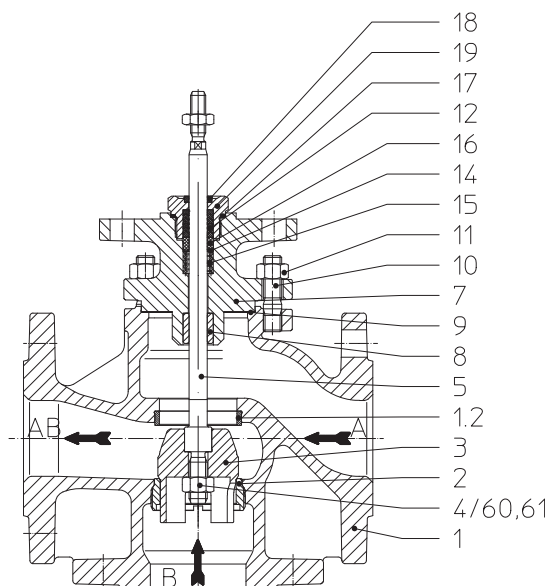
Рис. 1: BR 450 DN15-150
