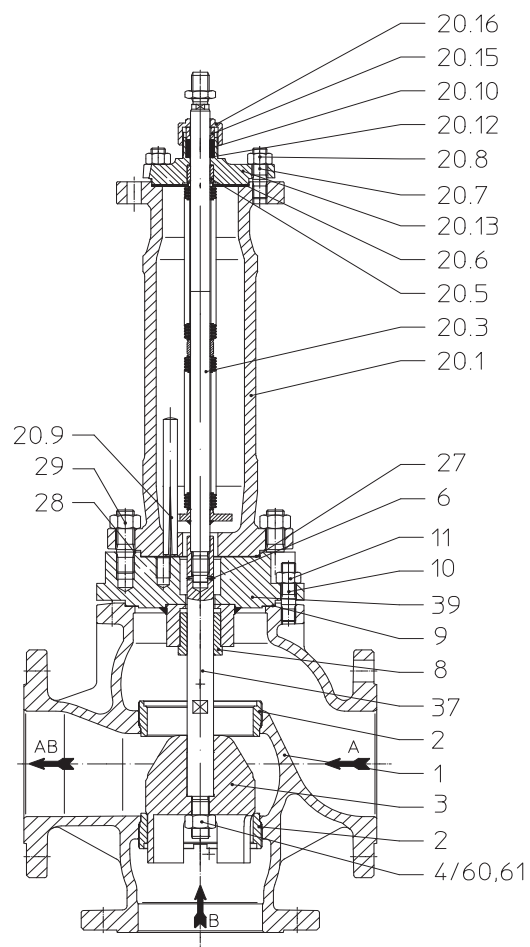
Рис. 4: BR 451 DN125v-150v
