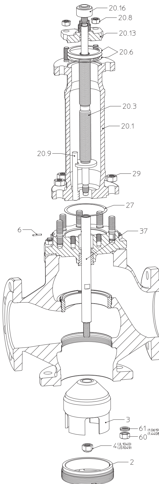
Рис. 17: BR 451 DN125v-150v со смесительным затвором
