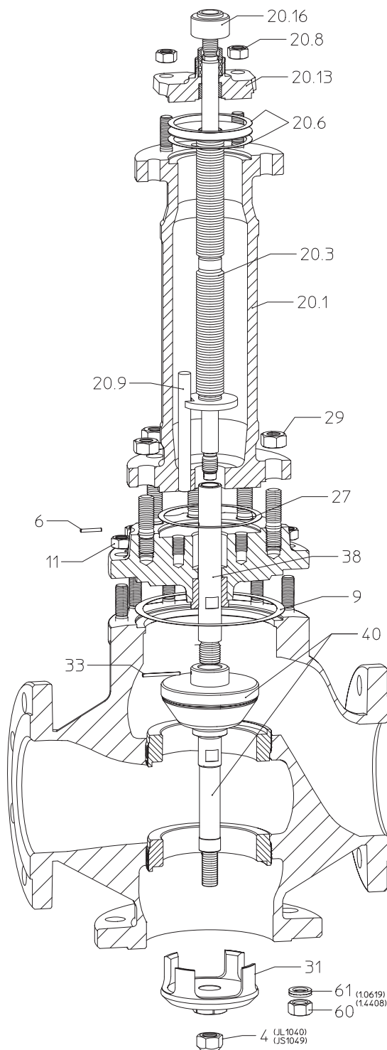
Рис. 19: BR 451 DN125v-150v с распределительным затвором
