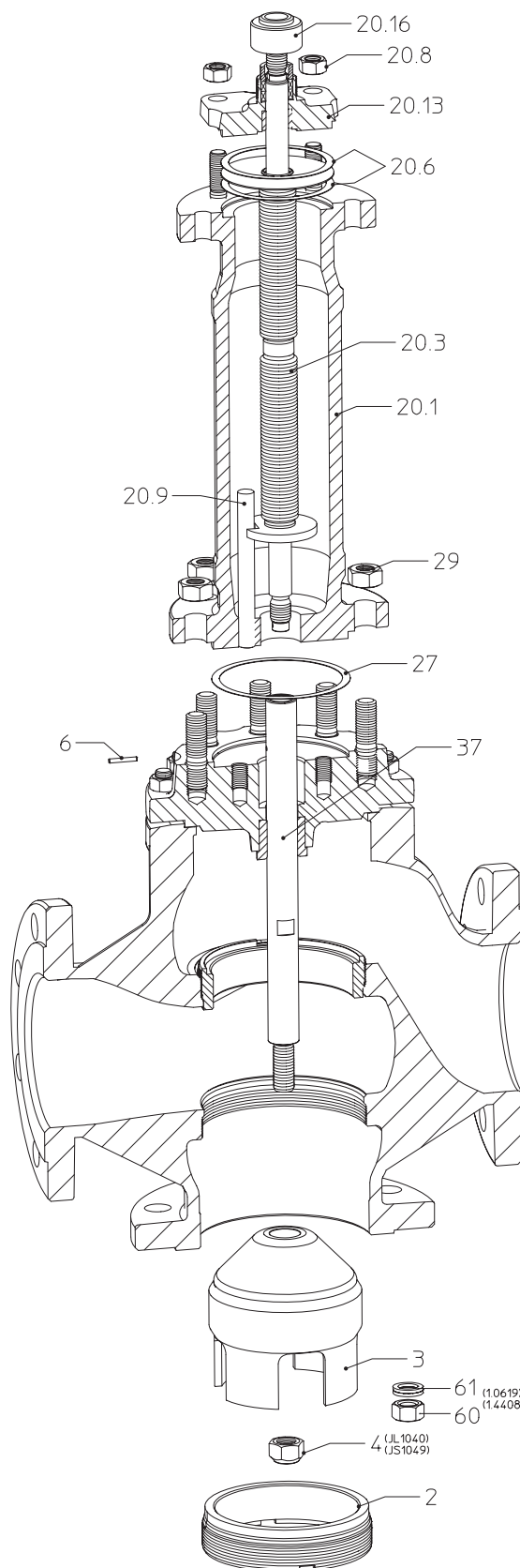
Bild 19: BR 451 DN125v-150v mit Mischkegel
