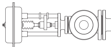
Bild 11: Rohrleitung waagrecht
