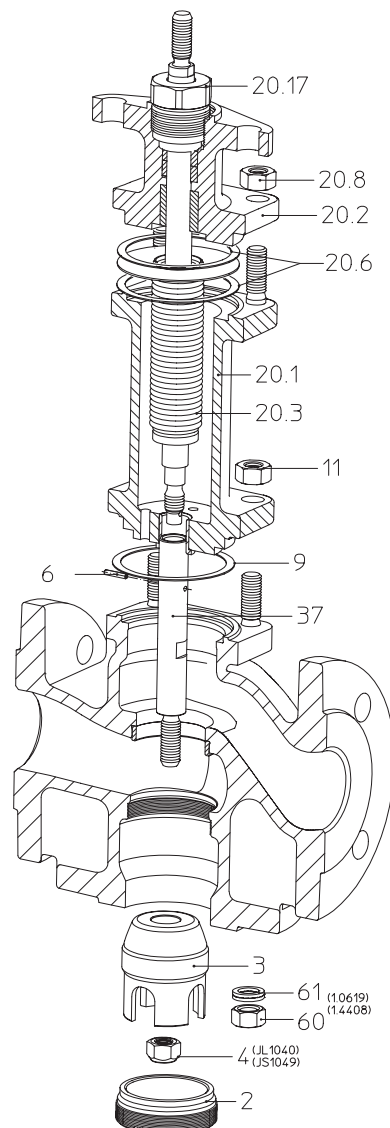
Bild 18: BR 451 DN 15-150 mit Mischkegel
