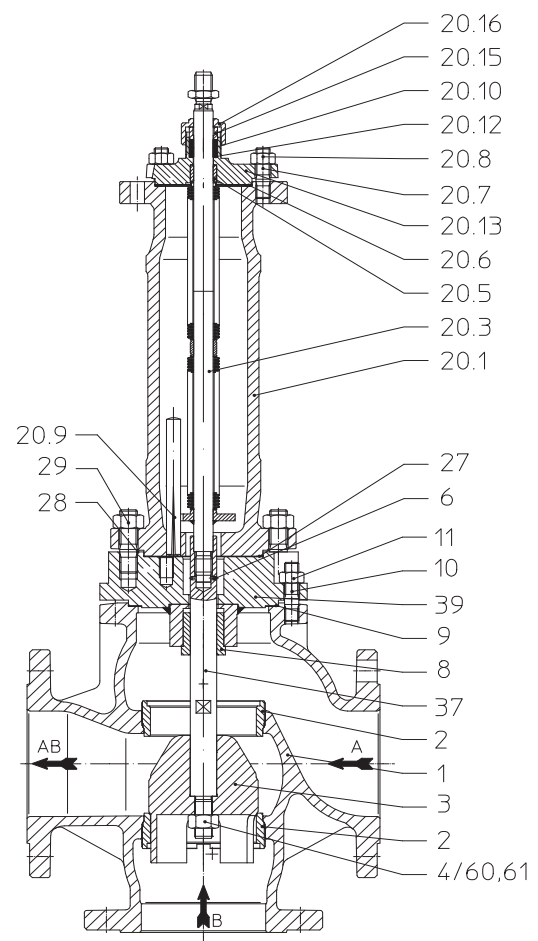
Bild 4: BR 451DN125v-150v
