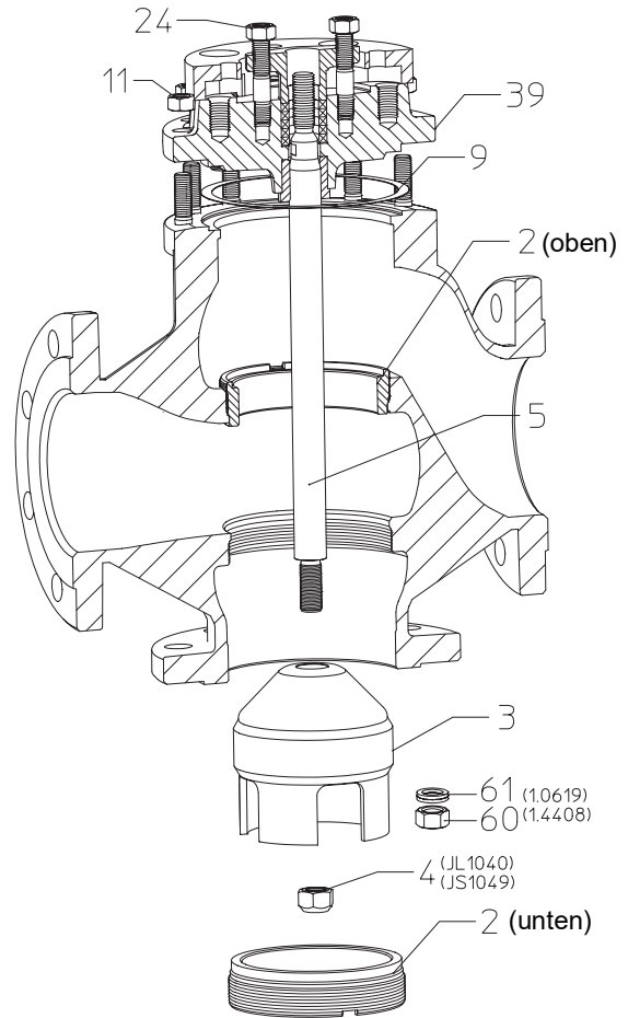
Bild 23: BR450 DN125v-150v mit Mischkegel
