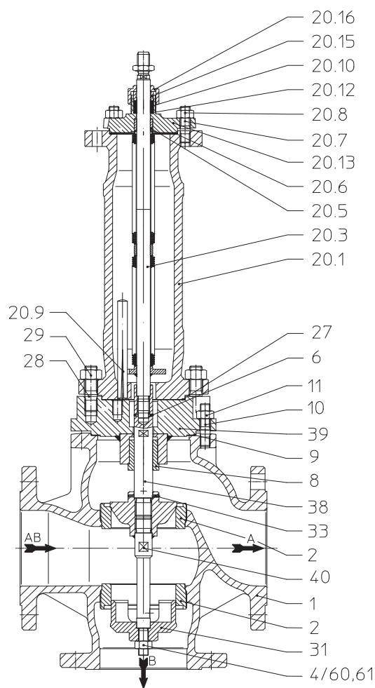
Bild 8: BR 451 DN125v-150v
