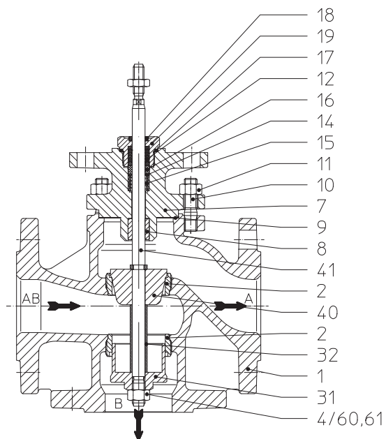
Bild 5: BR 450 DN15-150
