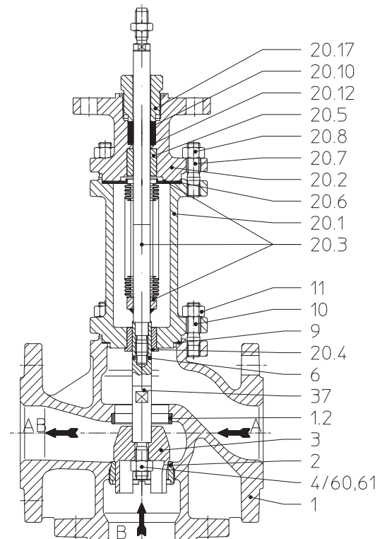
Bild 2: BR 451 DN15-150
