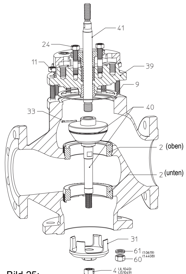
Bild 25: BR450 DN125v-150v mit Verteilkegel
