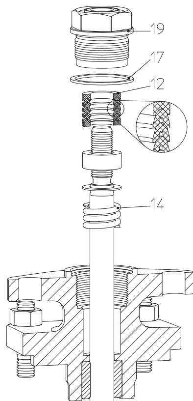
Bild 12: Dachmanschetten DN15-150
