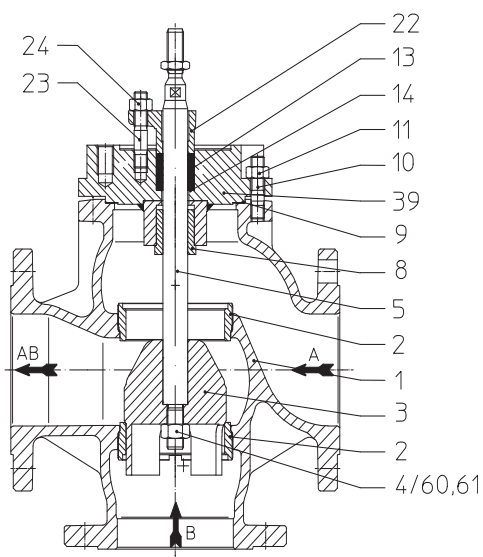
Bild 3: BR 450 DN125v-150v
