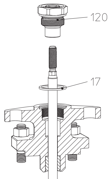
Bild 13: EPDM Abdichtung DN15 - DN150
