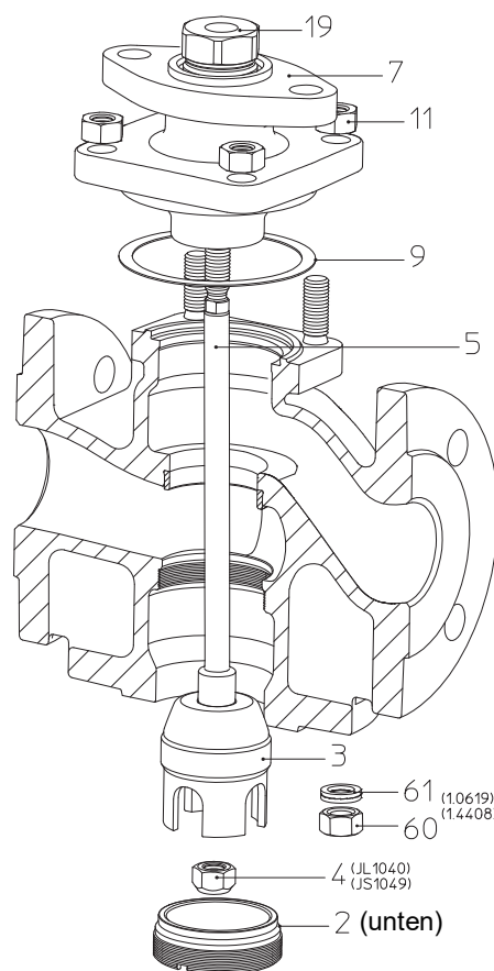
Bild 22: BR450 DN15-150 mit Mischkegel
