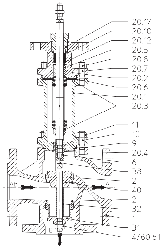
Bild 6: BR 451 DN15-150
