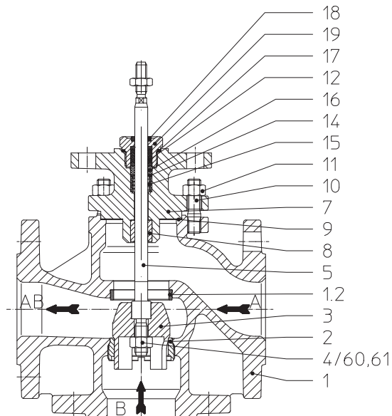
Bild 1: BR 450 DN15-150
