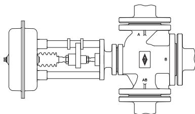
Bild 10: Rohrleitung senkrecht
