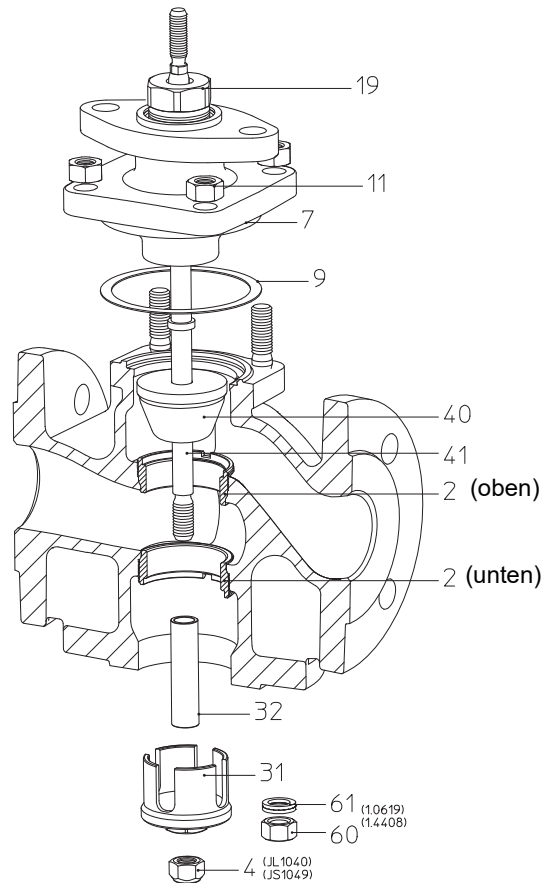
Bild 24: BR450 DN40-150 mit Verteilkegel
